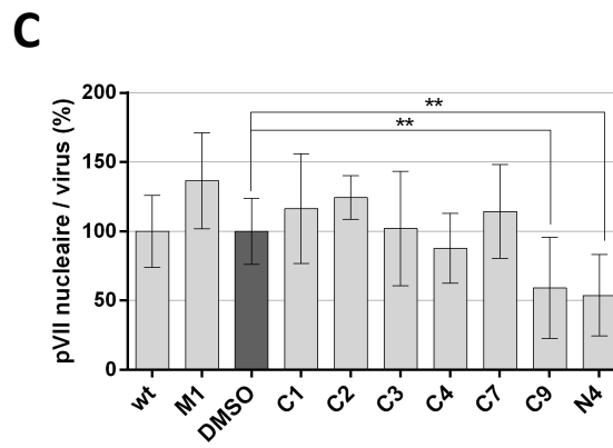
Figure 15: Effet des composés sur l'import nucléaire du génome de l'AdV. Nombre de protéine VII liée au génome viral dans les noyaux de cellules U2OS infectées avec 2500 pp/cellule de virus marqué Ad5-A488 (ou M1 lorsque précisé) pendant 2 h en présence de 5 \mu M des composés C1 à C9, 1 \mu M du composé N4 ou de DMSO comme contrôle. (A) Exemple d'images d'immunofluorescence avec les virus marqués ( en vert ), les protéines VII ( en rouge ) et le noyau marqué par du DAPI. Après immunomarquage des protéines VII, (B) le nombre de protéines VII nucléaires a été déterminé et est représenté en nombre absolu de protéine VII par noyau, dans une population de plus de 10 cellules par condition, et (C) le nombre de protéine VII par noyau a été normalisé en fonction du nombre de virus fluorescents par cellule. L'ensemble des valeurs obtenues a été normalisé en fonction du contrôle DMSO seul.
