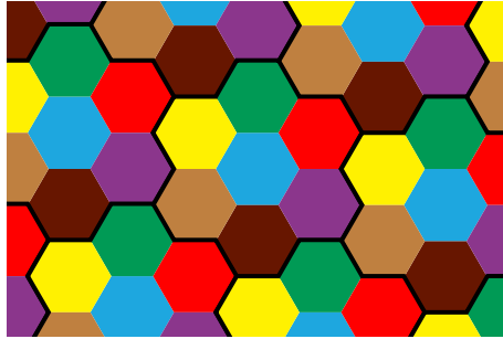
FIGURE 3. \chi(\mathbb{R}^2, \|\cdot\|_2) \leq 7 .
