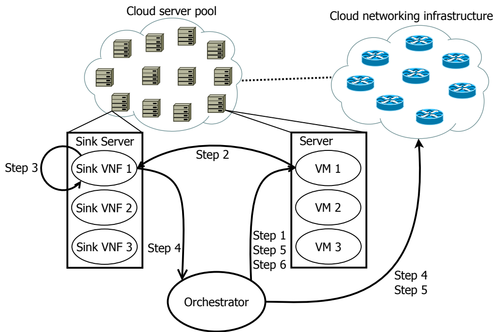
Figure 0.9: Procédure de migration d'une machine virtuelle à un Sink Server
