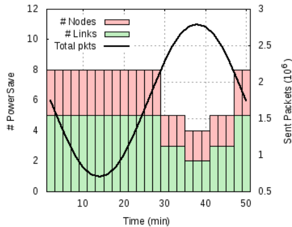
Figure 0.8: Numéro des liens/nœuds éteint en fonction du numéro des paquets envoyé pour atlanta.
