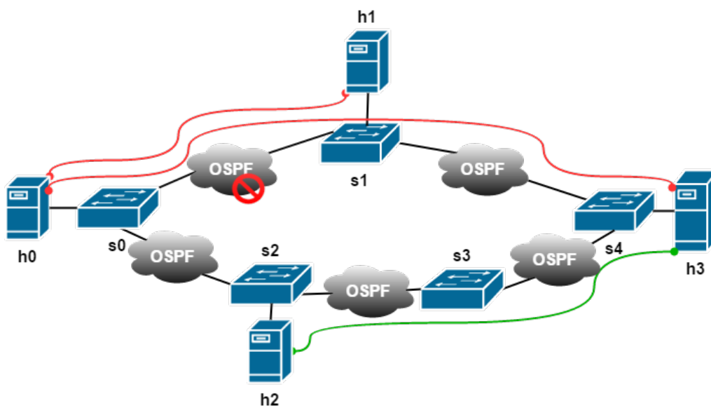
Figure 0.7: Réseau de teste PROPHYS.
