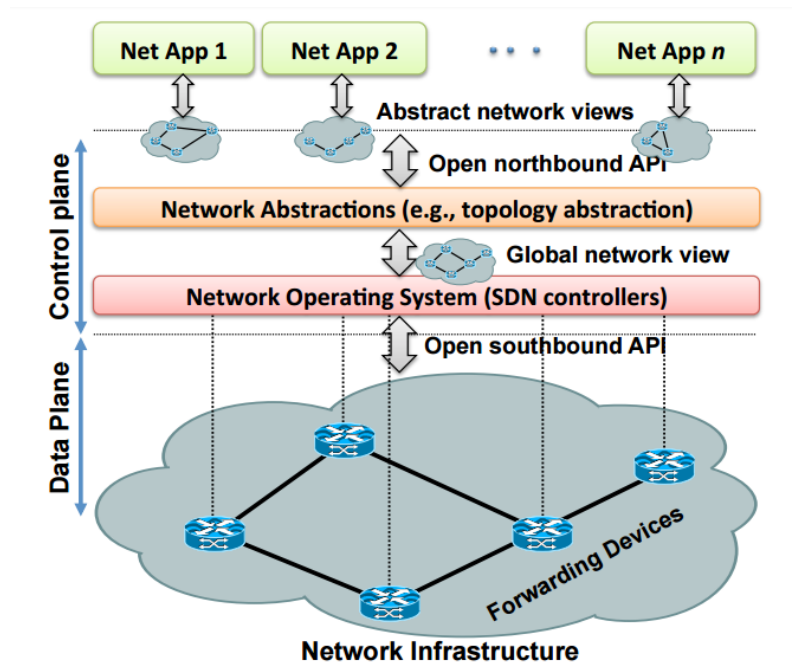
Figure 0.2: Structure de réseau basé sur SDN [KREV + 15]
