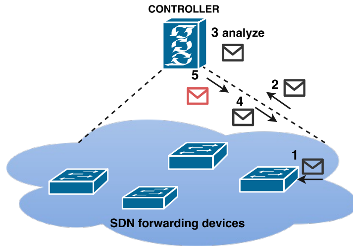
Figure 0.1: Traitement des paquets dans un réseau SDN.
