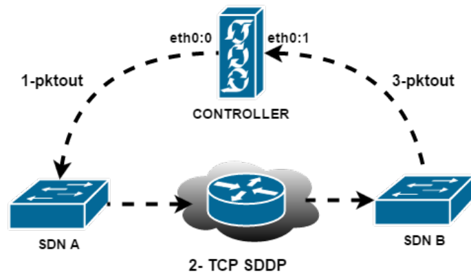
Figure 0.6: Transmission d'un paquet sonde de suivi du chemin issu du contrôleur.
