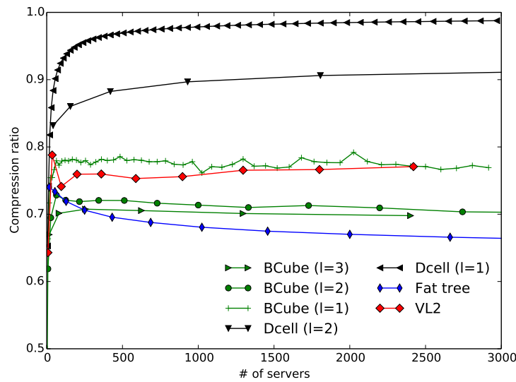
Figure 0.3: Taux de compression de MINNIE.
