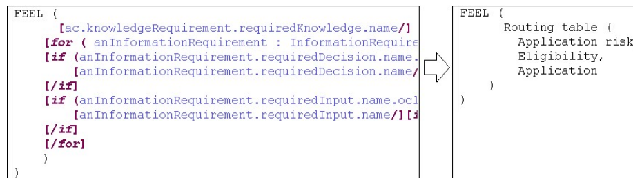
Figure 58 : Transformation Model-To-Text (FEEL) avec le module Acceleo
