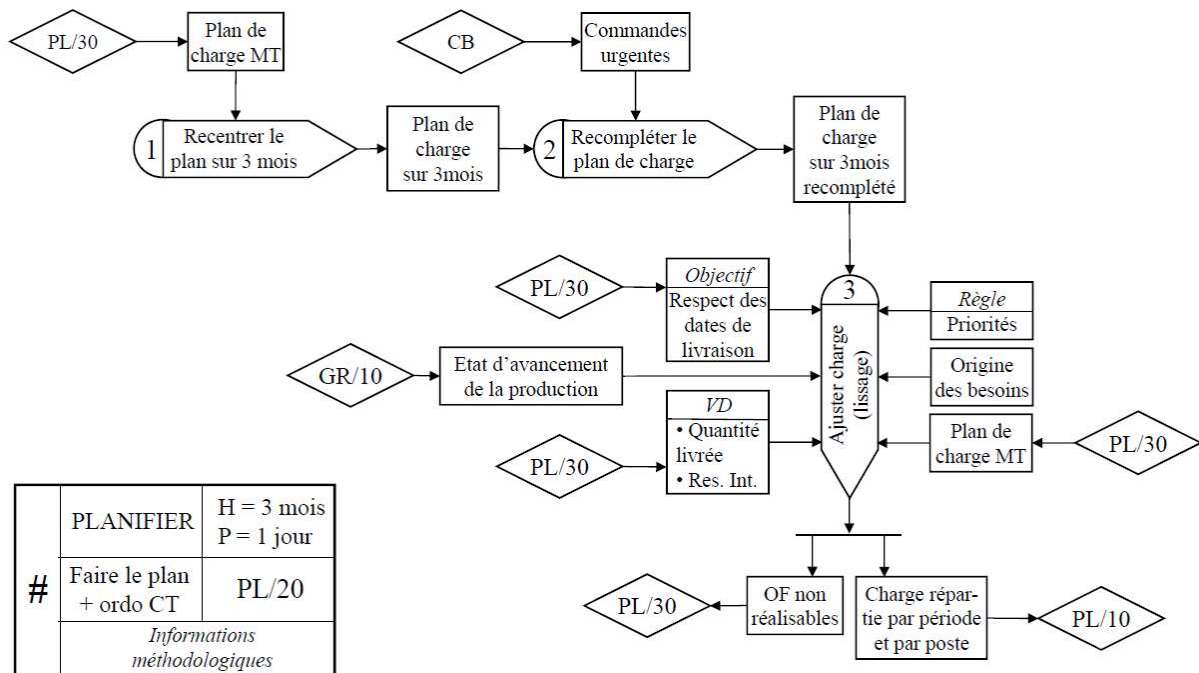
Figure 37 : Réseau GRAI pour Activité d'Exécution et Activité de Décision (Exemple)
