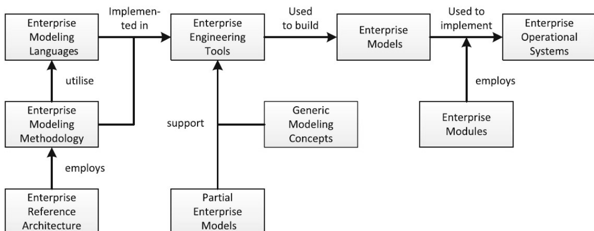
Figure 9 : Aperçu des composants de GERAM
