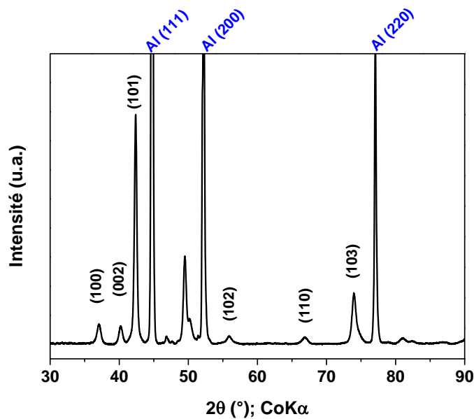
Figure IV. 5. Diffractogramme RX (Anode en Co) d'un film de ZnO déposé à partir d'une solution 0,1M de nitrate de zinc sur substrat d'aluminium, sous plasma Ar/O 2 , avec une température substrat de 200°C et une puissance plasma de de 300W.
