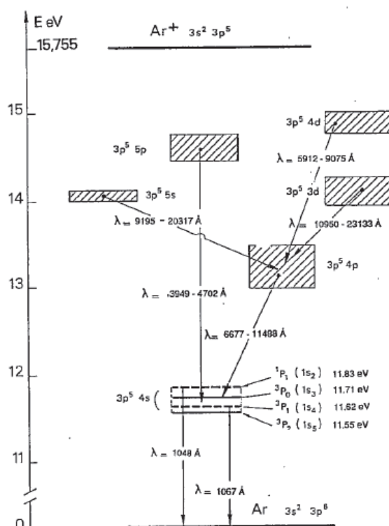
Figure III. 1. Diagramme des niveaux d'énergie de l'argon [10].
