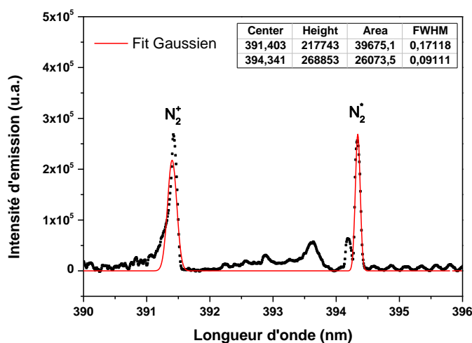
Figure III. 16. Fit gaussien obtenu sous Fytik® pour les raies N_2^+ à 391,4 nm et N_2^* à 394,3 nm.
