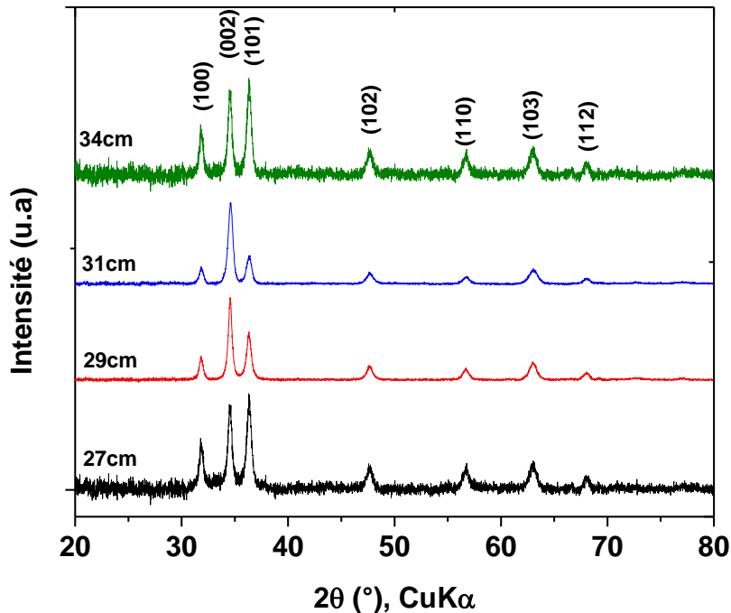
Figure IV. 7. Diffractogrammes RX de couches de ZnO déposées sur verres à différentes distances injecteur-substrat. Effet de la distance injecteur-substrat - \text{Zn}(\text{NO}_3)_2 0,2M (3 at % Al), 100% Ar; 300W; T_{\text{sub}}=200^\circ\text{C}
