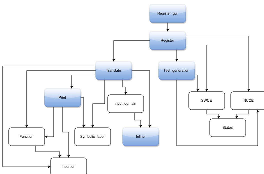
FIGURE 10.1 – Dépendances entre les modules de STADY
