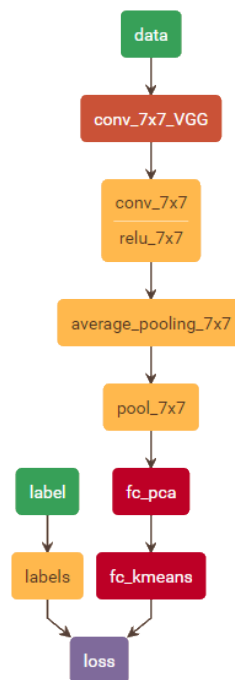
FIGURE 4.9 – Architecture de partitionnement.
