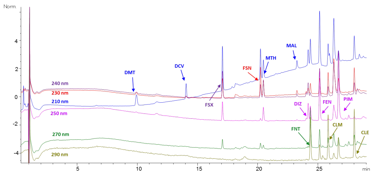
Figure 1. Séparation des OP à 1 mg/L en ACN a 210,230, 250,270 et 290 nm par LC-UV.
