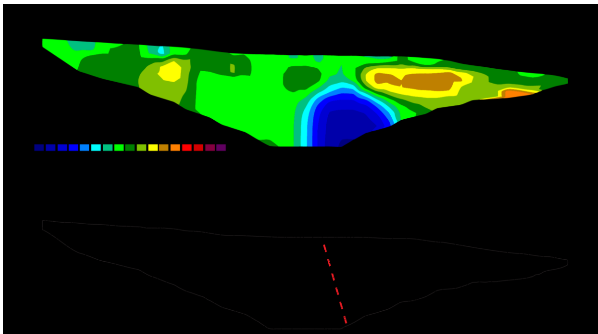
Figure III-35 : Profil électrique d localisé sur la Figure III-16, ainsi que son interprétation. L'espaceur inter-électrode est de 20 mètres. La configuration est Wenner-Schlumberger.
