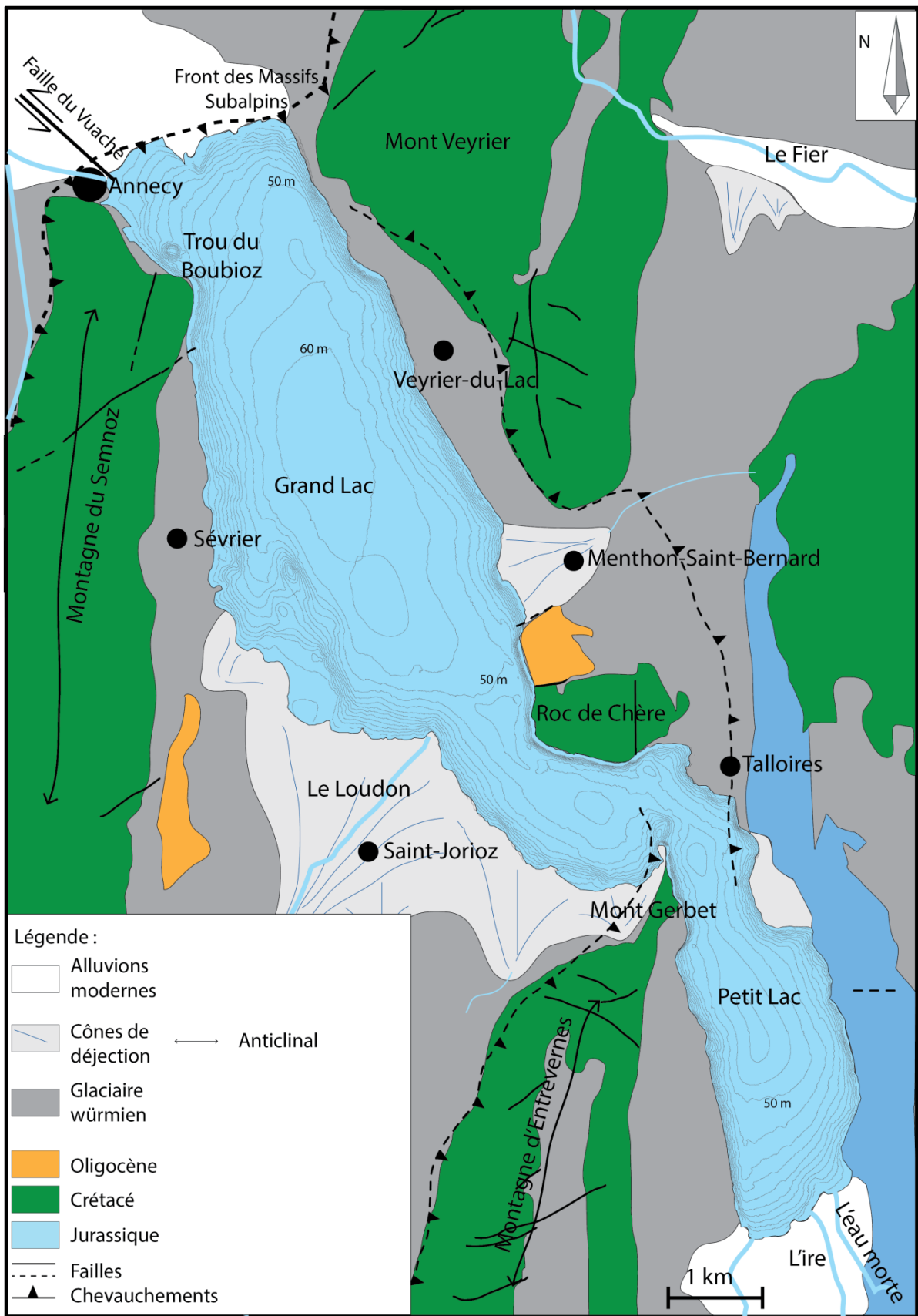
Figure I-35 : Schéma structural du Lac d'Annecy.
