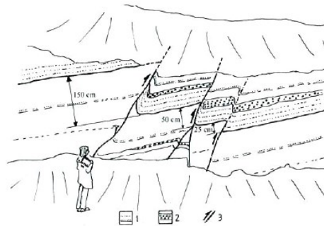
Figure I-9 : Coupe interprétée des séries fluvioglaciales de Saint Etienne de Crossey illustrant les déformations inverses les affectant de Baize et al. (2002). 1 : bancs-repères sableux ; 2 : niveaux de galets ; 3 : failles inverses.
