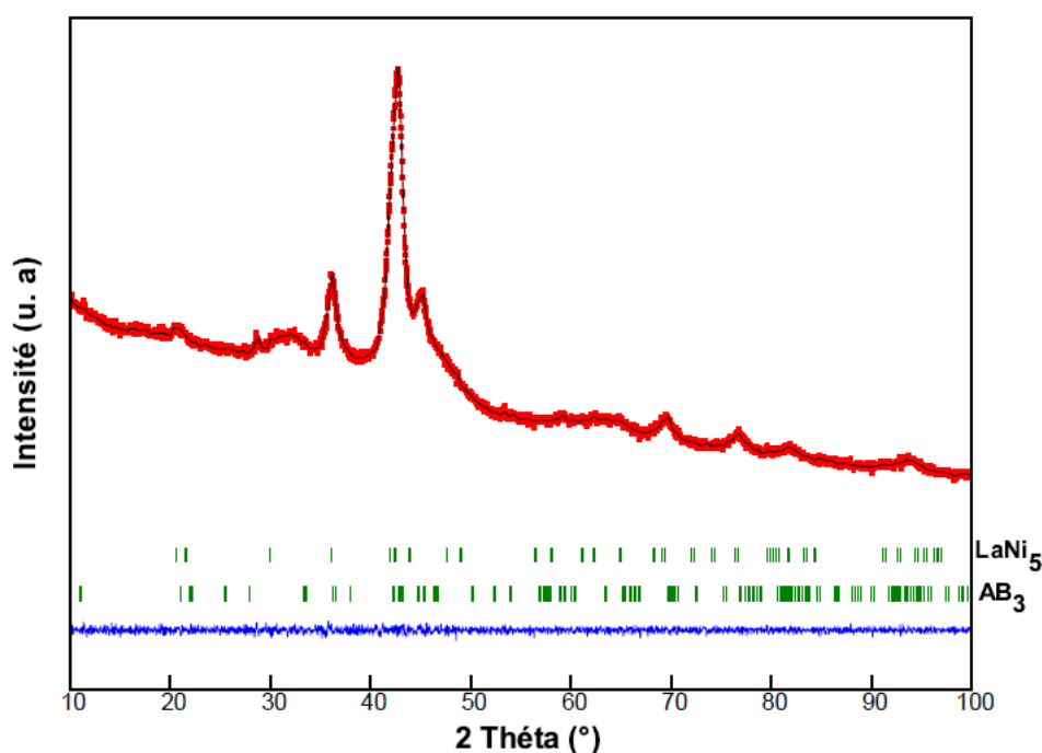
Figure III. 30: Affinement du diffractogramme de l'échantillon LCMN-M'10-P3 obtenu par mécanosynthèse ( \Delta t = 10\text{h} , P = 3.791\text{ W/g} ) à partir du mélange de poudres de \text{LaNi}_5 , \text{MgNi}_2 , Ca et Ni.
