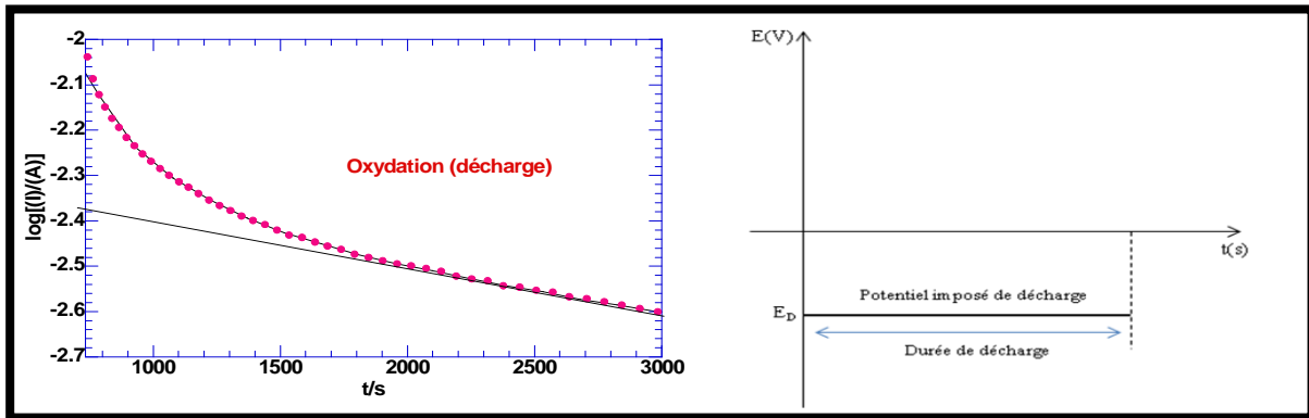
Figure II.18 : Potentiel de décharge imposé et chronoampérogramme correspondant.
