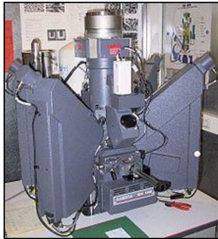
Figure II.9 : Microsonde électronique, modèle CAMECA SX 100.
