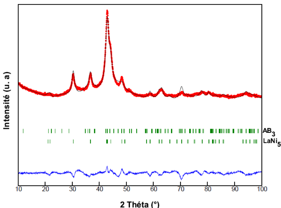
Figure III.42 :Affinement du diffractogramme de l'échantillon LCMN-M'10 obtenu par mécanosynthèse ( \Delta t = 10h , P = 4.135 W/g ) à partir du mélange de poudres de LaNi_5 , MgNi_2 , CaNiH_3 et Ni.
