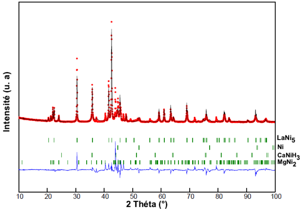
Figure III.41 : Affinement du diffractogramme de l'échantillon LCMN-M''0- obtenu par mécanosynthèse ( \Delta t = 0h , P = 4.135 W/g ) à partir du mélange de poudres de LaNi 5 , MgNi 2 , CaNiH 3 et Ni.
