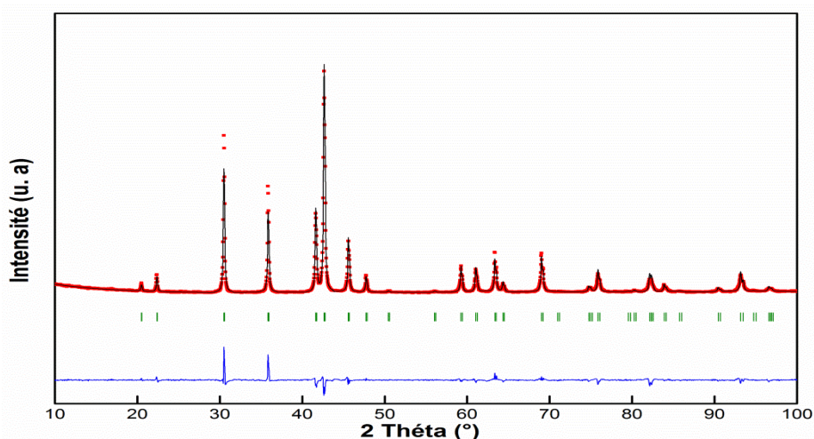
Figure III.23 : Diffractogramme de RX affiné du composé \text{LaNi}_5 obtenu par le four UHF.
