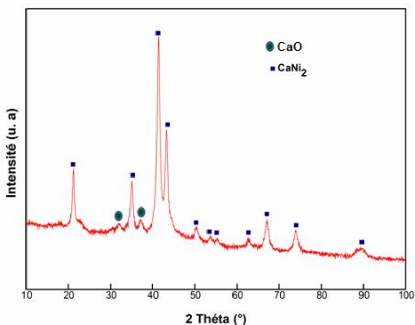
Figure III. 28: Diffractogramme de l'alliage CaNi 2 élaboré après 40 h de mécanosynthèse.
