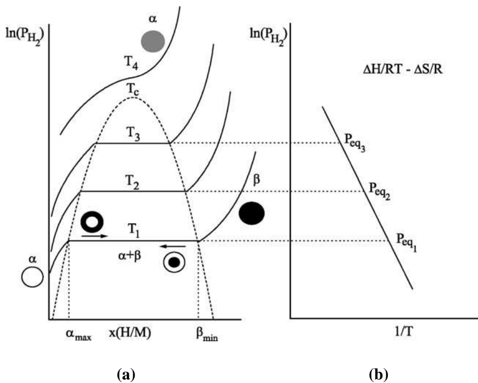
Figure I. 2: (a) Courbes P-C-T à différentes températures pour un même matériau dans le cas idéal. (b) variation de \ln[P(H_2)] en fonction de 1/T en relation avec la loi de Van't Hoff [1].
