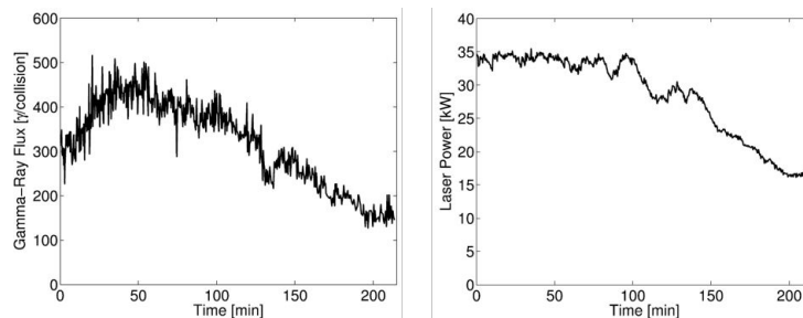
Figure 6.18: Gauche : évolution du flux de rayons \gamma en fonction du temps pour l'expérience MightyLaser. Droite : évolution de la puissance stockée correspondante. Images tirées de la Ref. [48].
