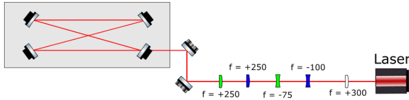
Figure 5.8: Définition du télescope. En blanc la lentille sphérique, en bleu les lentilles agissant dans le plan tangential, en vert les lentilles pour le plan sagittal. Les valeurs sont en mm.
