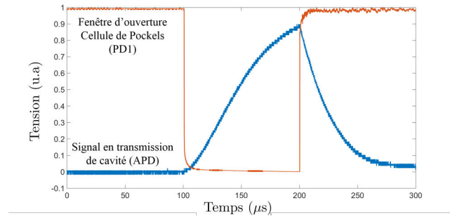
Figure 4.5: Exemple de signaux expérimentaux avec en bleu la transmission de la cavité pour t_p = 100 \mu\text{s} et en rouge le temps d'ouverture de la cellule de Pockels.
