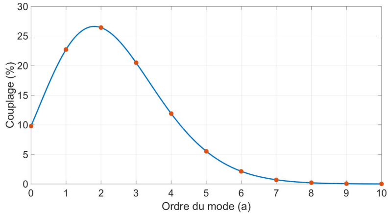
Figure 5.3: Couplage aux modes transverse d'une cavité optique d'un faisceau ayant un défaut angulaire de 0.5 mrad, une taille de waist de 1 mm et \lambda_0 = 1030 nm. Le couplage est mesuré au waist de la cavité. En bleu la distribution de Poisson associée au couplage.
