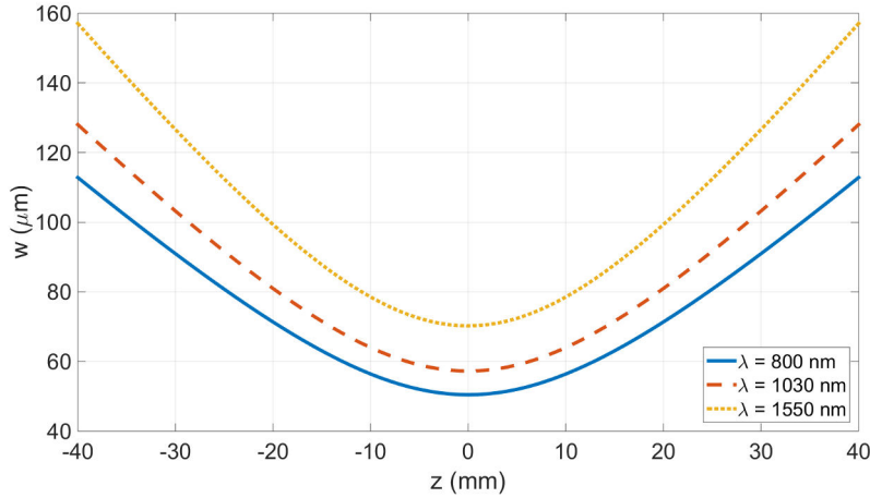
Figure 2.4: Evolution de la taille transverse d'un faisceau gaussien "iso-diffracting" pour différentes longueurs d'onde, avec a = 20 mm. A partir de l'Eq. 2.27.
