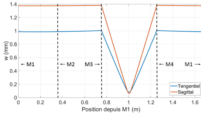
Figure 3.5: Variation de la taille transverse du faisceau le long de la propagation dans la cavité P178-a.
