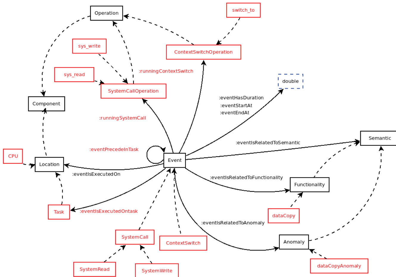
Figure 3.1: Extrait des classes et propriétés de VIDCOM pour l'analyse de la trace exemple
