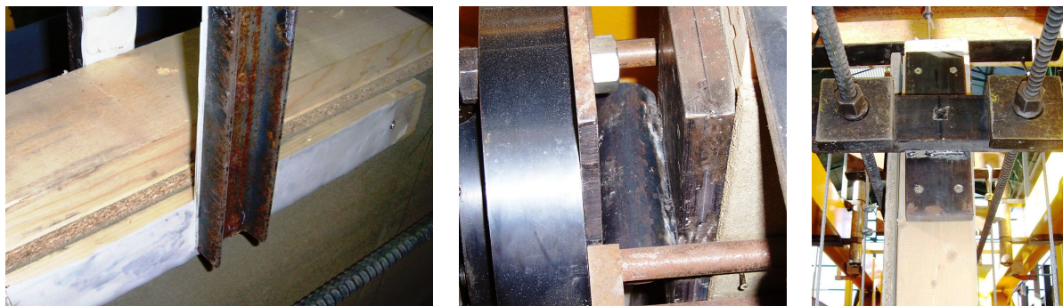
(a) Glissière
