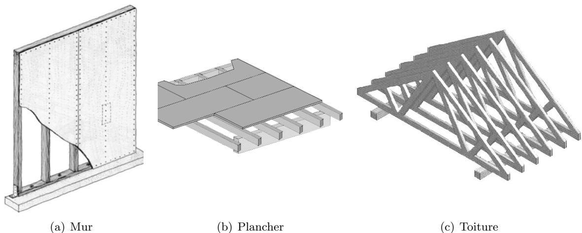
Figure 6.1: Éléments de structure à ossature bois
