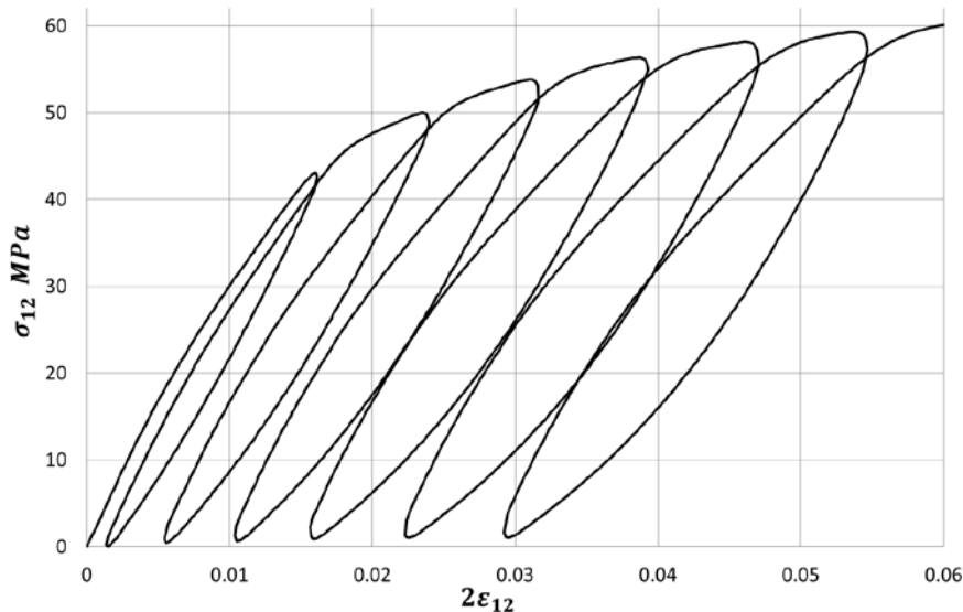
Figure 4.9. Courbe contrainte/déformation de cisaillement à 50 mm/min pour composite à matrice thermdurcissable
