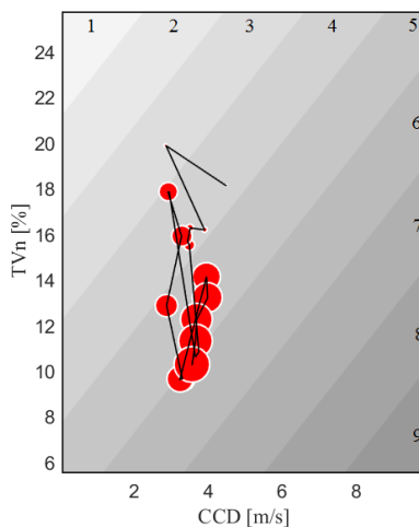
Figure 44 - Exemple d'une évaluation systématique d'une méthode de partitionnement
