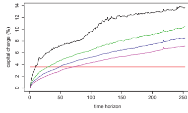
Figure 2.40: PCA CC
