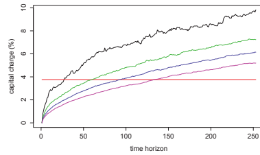
Figure 2.43: PCA CC
