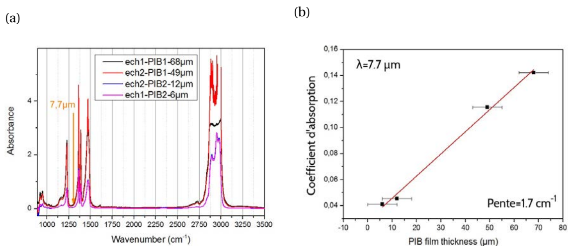
FIGURE 3.37 – (a) Spectre d'absorption du PIB dans le MIR. (b) Absorption du PIB en fonction de l'épaisseur de la couche à 7.7 µm.
