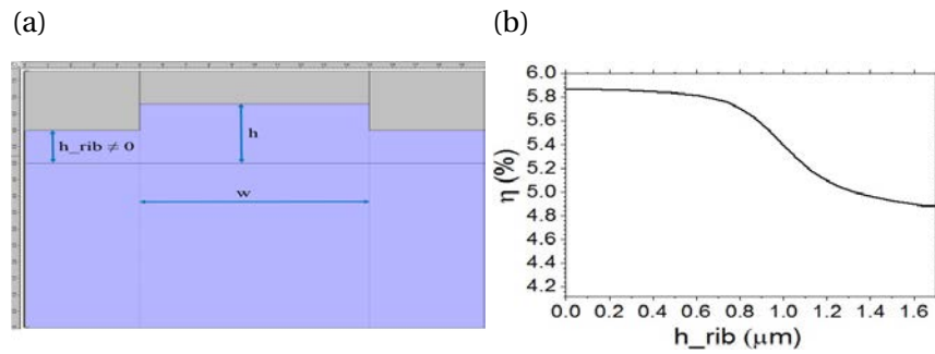
FIGURE 3.25 – (a) Géométrie d'un guide rib. (b) Évolution du facteur de champ évanescent en fonction de l'épaisseur h_{rib} calculée pour un guide rib de dimensions w=10 \mu m , h=1.8 \mu m à \lambda=7.7 \mu m pour la polarisation TM.
