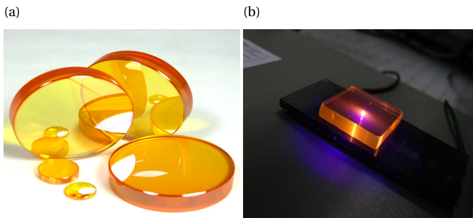
FIGURE 2.2 – Exemples de photographies de verres de chalcogénure : (a) Séléniure [177]. (b) Tellure [178].
