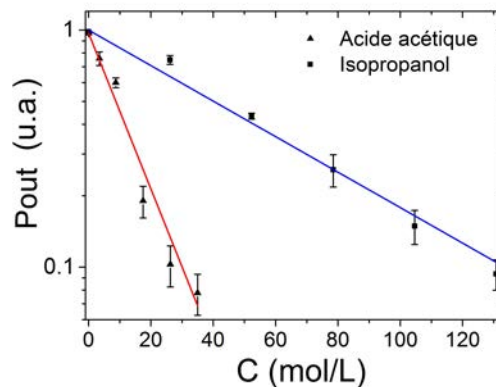
FIGURE 4.17 – Évolution de la réponse du capteur optique intégré en fonction des concentrations de l'isopropanol et l'acide acétique en mol/L à 7.7\ \mu\text{m} .
