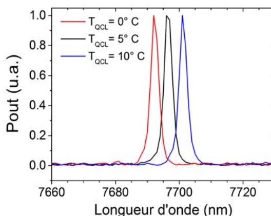
FIGURE 2.25 – Caractérisation spectrale du QCL en fonction de la température interne de la puce.
