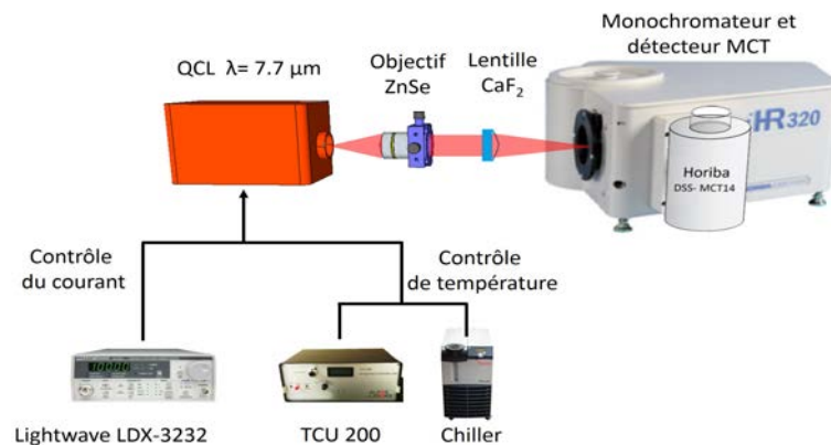
FIGURE 2.24 – Configuration expérimentale pour la caractérisation spectrale du QCL en fonction de la température interne de la puce.
