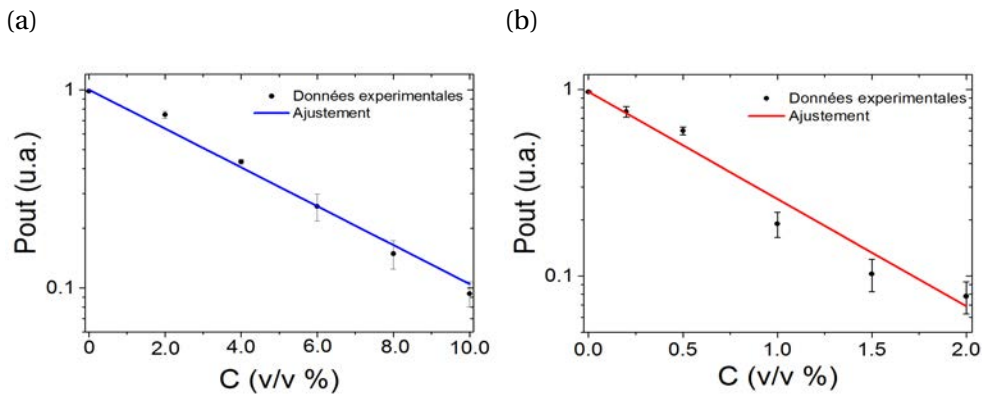
FIGURE 4.16 – Réponse du capteur optique intégré en fonction des différentes concentrations de (a) l'isopropanol et (b) l'acide acétique en pourcentage volumique à 7.7\ \mu\text{m} .
