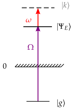
FIGURE 5.1: Ionisation à deux photons XUV-IR depuis l'état initial vers un état du continuum via une résonance d'auto-ionisation.
