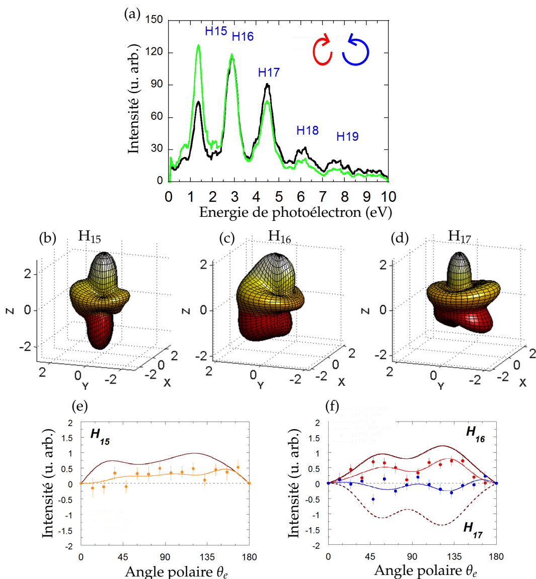
FIGURE 14.10: Polarimétrie moléculaire dans le cas \epsilon_{\text{IR}} \approx +0.84 ; \epsilon_{\text{UV}} \approx -1 . (a) Spectre de photoélectrons issu de la PID de NO mesuré (noir) et corrigé de la section efficace du processus (vert). (b-d) DAPRM réduites I(\theta_e, \phi_e) lorsque la molécule de NO est perpendiculaire à la direction de propagation du faisceau pour les harmoniques 15, 16 et 17. (e-f) Produit s_3 \times F_{11}(\theta_e) mesuré pour H 15 (orange), H 16 (rouge) et H 17 (bleu) (points expérimentaux avec leur barre d'erreur et ajustement en polynômes de Legendre), et fonctions F_{11}(\theta_e) de référence mesurées au synchrotron (brun). Dans cette gamme d'énergie, les F_{11} sont positives, cependant pour mettre en évidence le signe de s_3 la fonction de référence -F_{11}(\theta_e) est représentée dans les cas où s_3 < 0 .
