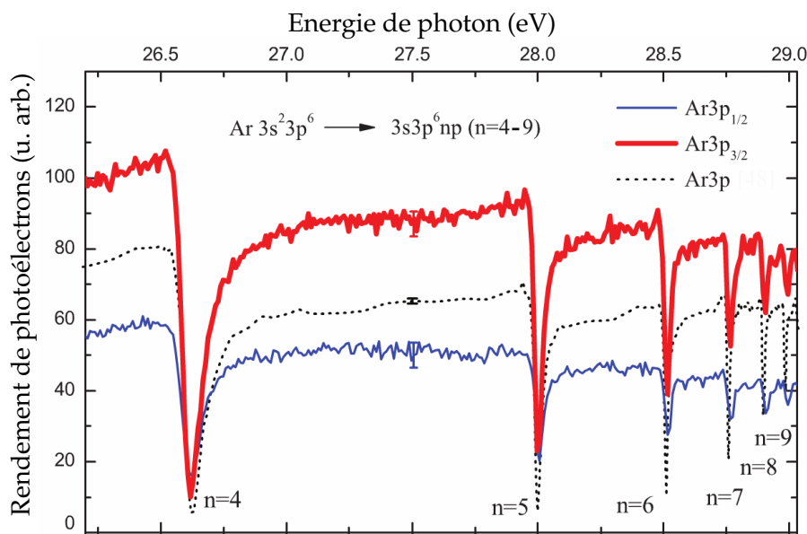
FIGURE 11.1: Rendement de photoélectrons résolu en spin-orbite au voisinage des résonances 3s^2 3p^6 \rightarrow 3s 3p^6 np ( n = 4 - 9 ) de l'argon. La ligne pointillée noire est une mesure non résolue en spin-orbite mais avec une meilleure résolution [Berrah et al., 1996]. Extrait de [Zhang et al., 2009].
