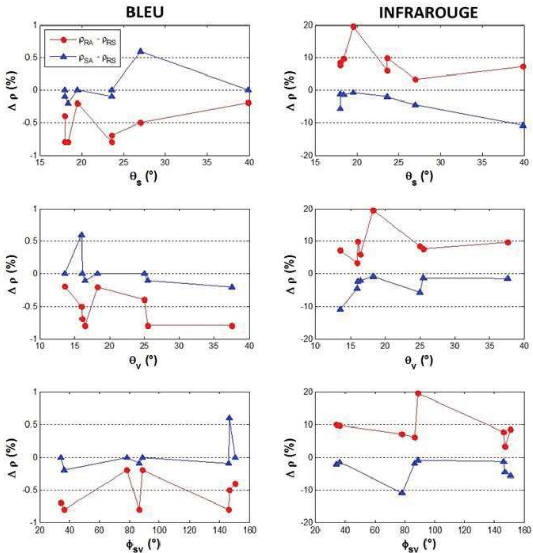
Figure 47: Différentiels de réflectance des zonations à RA et SA par rapport aux zonations à RS en fonction de \theta_s , \theta_v et \phi_{s-v} (domaine du bleu, à gauche, domaine du proche infrarouge à droite).
