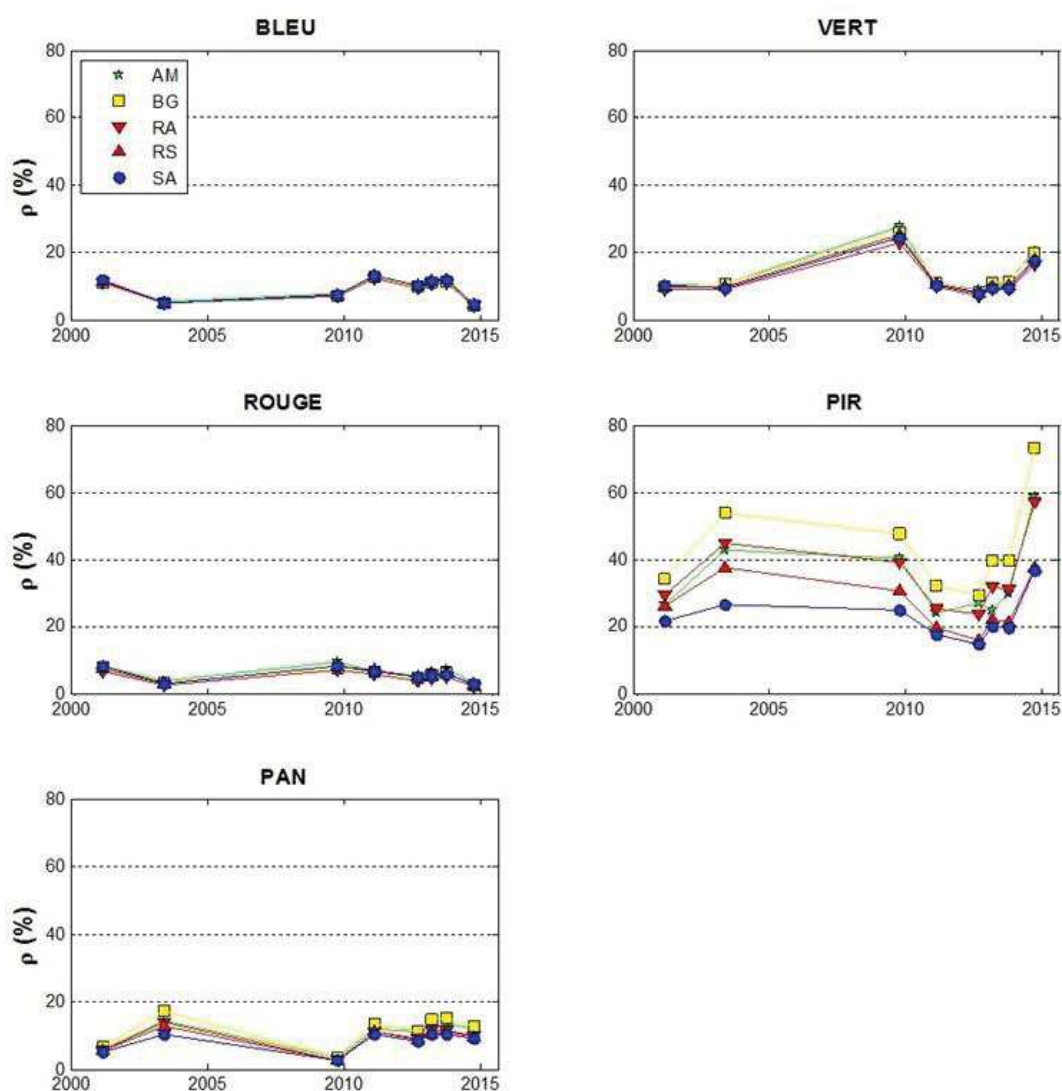
Figure 44: Variations temporelles des réflectances mesurées sur 5 formations de mangroves à forte mono-dominance pour 5 bandes spectrales.
