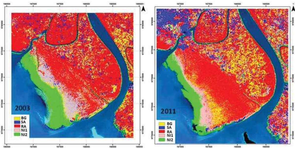
Figure 52: Cartographie à 5 espèces sur une région de Papoua Oueſt, région d'Inanwatan. Les espèces BG, SA et RA étaient facilement identifiables par comparaison avec Nusa Lembongan. Par contre, nous avons entraîné la classification sur 2 autres classes pour lesquelles l'espèce est sujette à caution. Les cartes font 2.5 km x 2.5 km.
