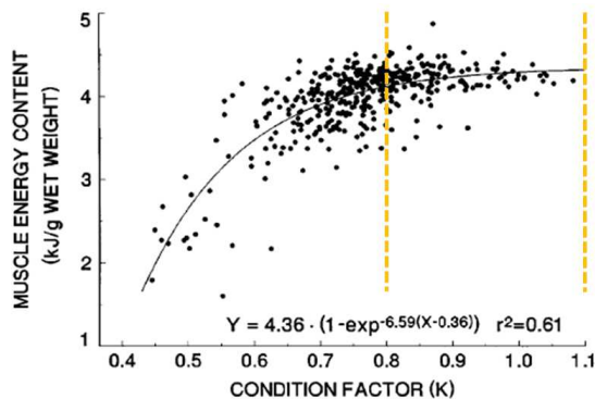
Fig. 9.2: Relation entre le contenu énergétique du muscle et l'indice de condition de Le Cren ( K_n ) chez la morue Gadus morhua observée par Lambert et Dutil (1997). Les pointillés orange figurent la gamme de variation de ce même indice observée chez les thons tropicaux dans notre étude.
