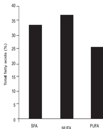
Figure B1 : Proportions des trois principales familles d'acides gras (SFA=Acides gras saturés; MUFA=Acides gras mono-insaturés; PUFA=Acides gras poly-insaturés) dans les lipides totaux du muscle de Diaphus wataesi , un myctophidé de la Mer d'Arabie – Sebastine et al. 2011
