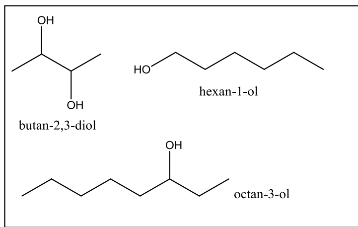
Figure 9. Structures de quelques alcools
