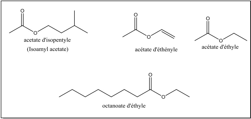
Figure 15. Structures de quelques esters
