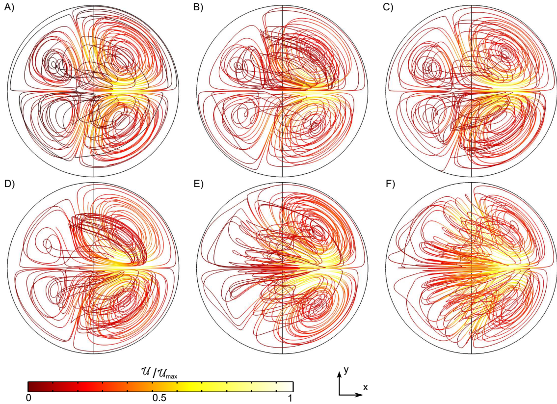
FIGURE B.6 : Lignes de courant des   coulements calcul  s avec les m  mes param  tres que les exp  riences de la figure B.6. La visualisation se fait par dessous. L'onde se propage de gauche    droite avec une amplitude u_0 = 44 pm. Le volume de la goutte est V_{goutte} = 12.5 \mu\text{l} . Nous retrouvons la transition de 4    2 vortex    mesure que la viscosit   augmente. (A) Eau pure ( U_{max} = 173 \mu\text{m/s} ) (B) 30 wt% Glyc. ( U_{max} = 170 \mu\text{m/s} ) (C) 40 wt% Glyc. ( U_{max} = 137 \mu\text{m/s} ) (D) 60 wt% Glyc. ( U_{max} = 61 \mu\text{m/s} ) (E) 80 wt% Glyc. ( U_{max} = 23 \mu\text{m/s} ) (F) 90 wt% Glyc. ( U_{max} = 3.8 \mu\text{m/s} ).
