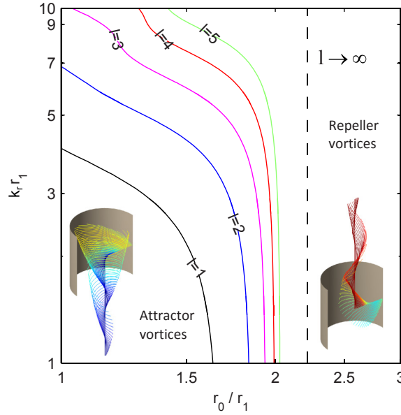
FIGURE B.11 : Lignes de niveau solutions de \bar{v}_z(r=0) = 0 pour différentes charges topologiques l , dimension typique k_r r_1 et ratio géométrique r_0/r_1 . L'espace des paramètres est divisé en deux domaines, l'un près de l'origine correspond aux vortex attracteurs avec une vitesse axiale négative en r=0 et l'autre correspond aux vortex répulsifs . La ligne en pointillé à r_0/r_1 \sim 2.218 indique une limite asymptotique pour les grandes valeurs de l .
