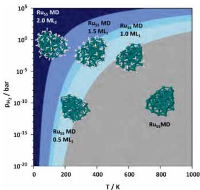
FIGURE 5.17: Diagramme de phase pour Ru 55 MD avec et sans hydrogène adsorbé.
