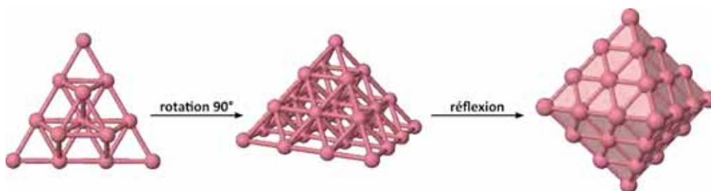
FIGURE 3.24: Construction de l'octaèdre à deux couches par rotation et réflexion.
