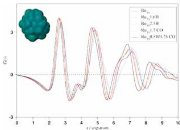
FIGURE 3.43: Profil RDF théorique d'un cluster \text{Ru}_{55} hcp avec espèces adsorbées à la surface. Les intensités sont données en unités arbitraires. ( \sigma_0 = 0.2 , \sigma_{BL} = 1.0 , A_{BL} = 0.045 , \delta = 0.02 , \gamma = 0.06 , \alpha = 0.025 )
