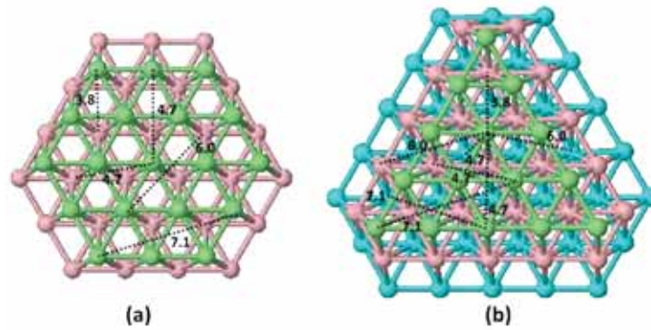
FIGURE 3.39: Distances standard dans un empilement (a) AB ou (b) ABC pour une distance interatomique de 2.7 \text{ \AA} . La couche A est représentée en vert, la B en rose et la C en bleu.
