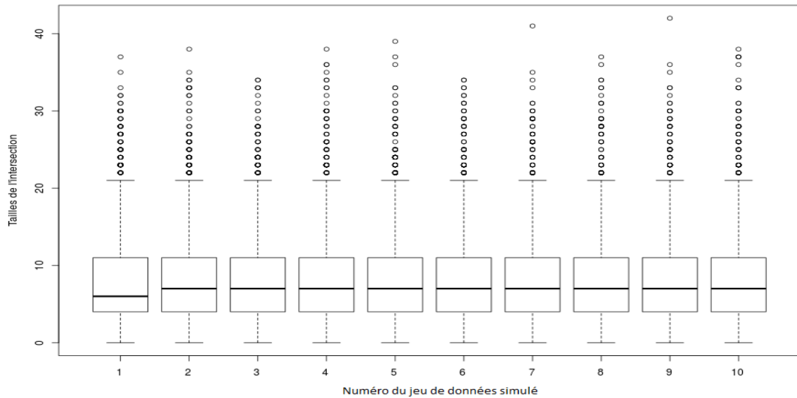
FIGURE 4.3 – Répartition de la taille de l’intersection, pour chaque jeu simulé s_k , entre les supports \{s_k S_j^{GLstab}\}_{j \in \{1, \dots, p\}} et les supports \{\widehat{S}_j^{GLstab}\}_{j \in \{1, \dots, p\}}
