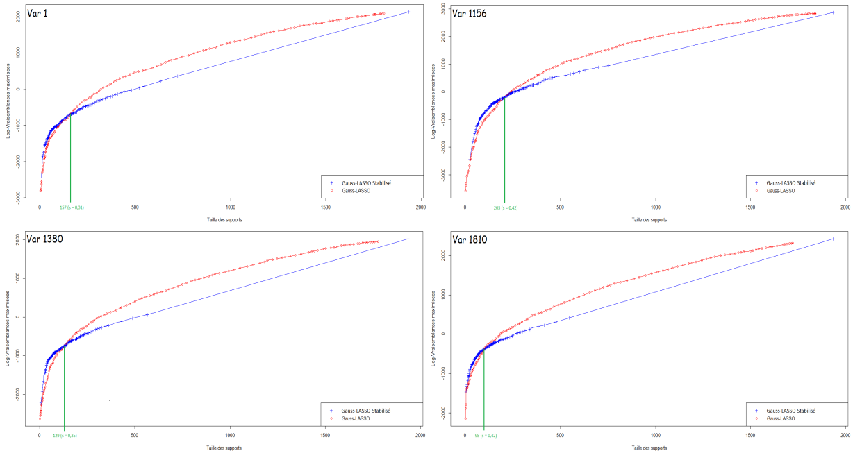
FIGURE 2.26 – Comparaison de l'évolution de V_{max} (M_j^{GLstab}(s_j)) et de V_{max} (M_j^{GL}(\lambda_j)) en fonction de la taille des support associés aux modèles pour 4 des variables typiques
