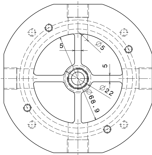
Vue de dessus Echelle : 1:1
