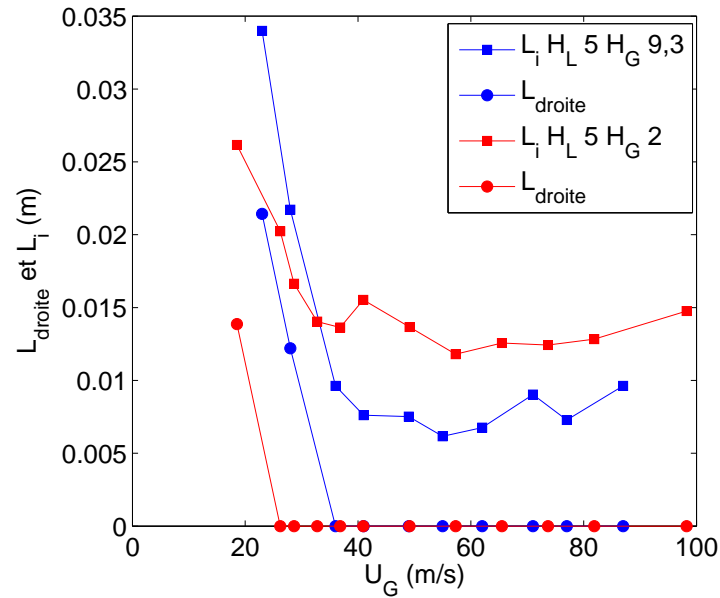
FIGURE 4.11 – Longueur droite L_{droite} et L_i fonction de la vitesse gaz pour l'injecteur n°2 H_L 5 \text{ mm } H_G 9.3 \text{ mm} , U_L = 0,42 \text{ m/s} (bleu) et H_L 5 \text{ mm } H_G 2 \text{ mm} , U_L = 0,42 \text{ m/s} (rouge).
