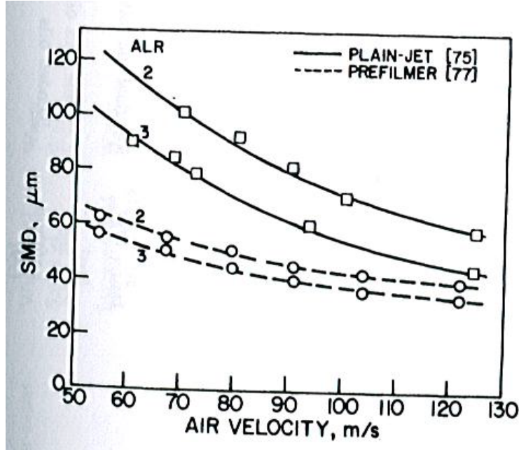
FIGURE 1.28 – Comparaison des tailles de gouttes moyennes pour la géométrie d'injection plane avec préfilmage et la géométrie d'injection coaxiale, Lorenzetto et Lefebvre 1977 [51].
