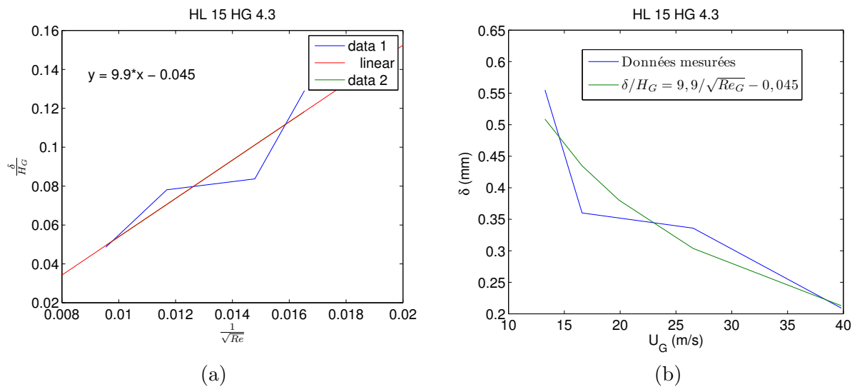
FIGURE C.5 – Épaisseur de vorticité H_L = 15 mm H_G = 4,3 mm.
