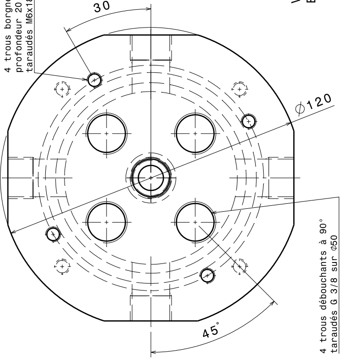
Vue de derrière Echelle : 1:1
