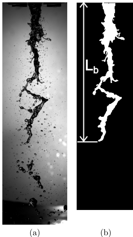
FIGURE 4.49 – Exemple d’image brute du jet (a) et d’image du jet extrait connexe (b), avec la mesure de L_b .
