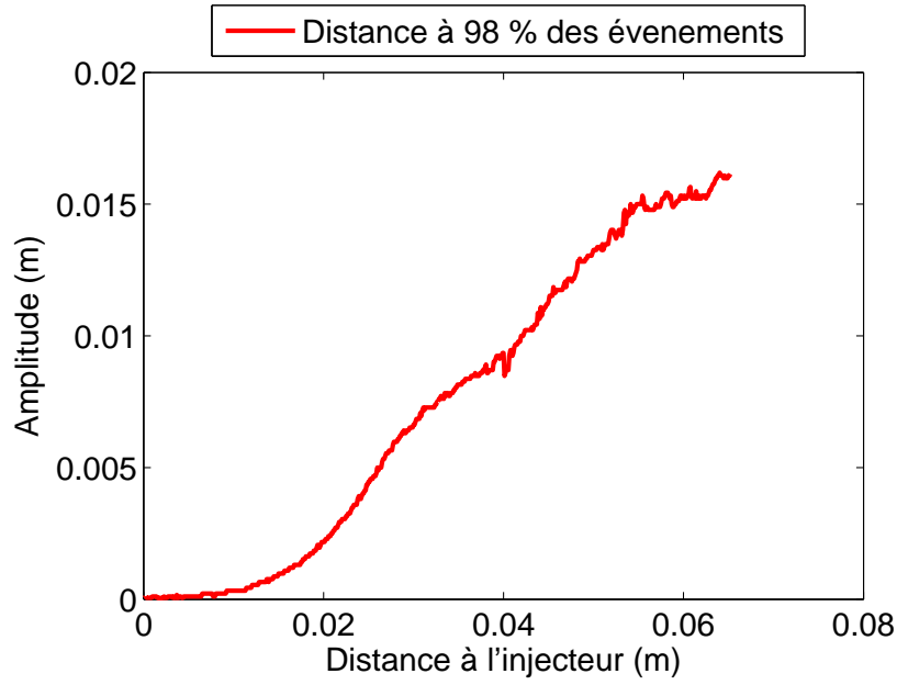
FIGURE 5.44 – Profil de l'amplitude du jet connexe à l'injecteur sans gouttes filtré et limité à 98 % des évènements (voir 4.2.1 pour les détails sur l'obtention de ce profil). Conditions expérimentales : injecteur n°2 H_L = 5 mm, H_G = 5 mm, U_L = 0,28 ms/s U_G = 19,5 m/s.
