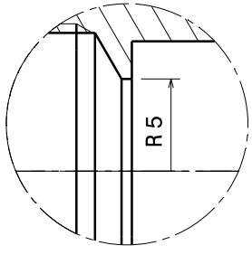
Détail I Echelle : 4:1
