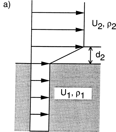
FIGURE 1.16 – Profil de vitesse de base utilis e pour l’analyse de stabilit  lin aire de Raynal 1997 [75].
