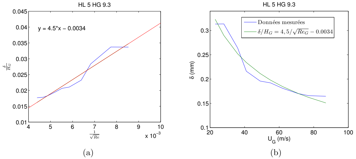
FIGURE C.3 – Épaisseur de vorticité H_L = 5 mm H_G = 9,3 mm.
