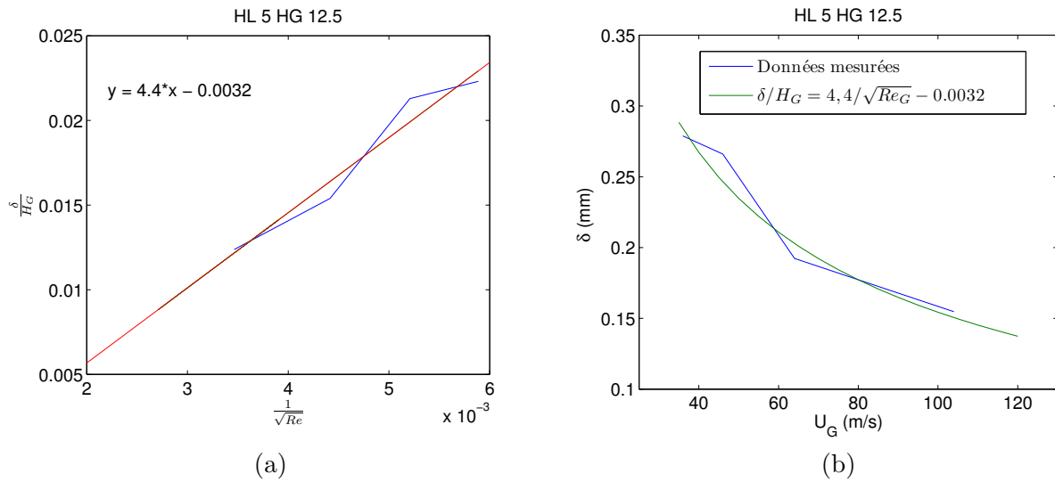
FIGURE C.4 – Épaisseur de vorticité H_L = 5 mm H_G = 12,5 mm.
