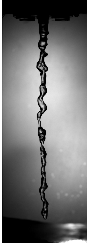
FIGURE 4.19 – Exemple de réalisation de jet pour l'injecteur n°2 H_L 20 mm H_G 1,8 mm U_L 0,23 m/s U_G 18 m/s.
