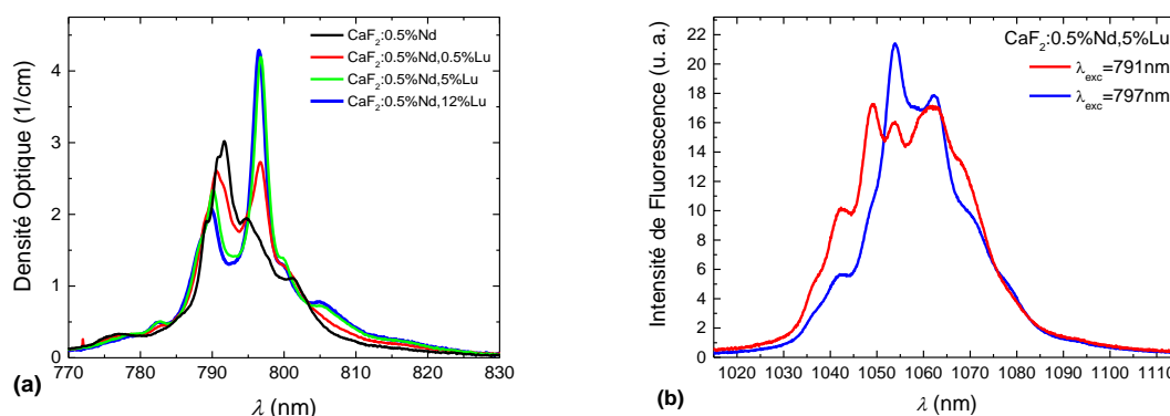
Fig. F4 (a) Spectres d'absorption CaF 2 :Nd 3+ ,Lu 3+ qui montrent les changements de forme de la bande avec l'incrément de la concentration du Lu 3+ . (b) Spectres d'émission de CaF 2 :0.5% Nd,5% Lu à différentes longueur d'onde d'excitation normalisés par la valeur du coefficient d'absorption à la longueur d'onde d'excitation correspondante. Le spectre à 791 nm montre une valeur d'aire intégrée comparable à celle du spectre à 797 nm.
