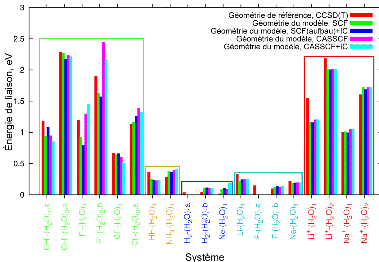
FIGURE 4.10 – Diagramme des énergies de liaison soluté-eau en fonction du soluté. Les énergies calculées avec le modèle correspondent aux énergies des géométries obtenues avec le modèle. Pour les énergies de référence CCSD(T), ces dernières correspondent aux énergies pour les géométries qui nous servent de référence, obtenues en CASPT2
