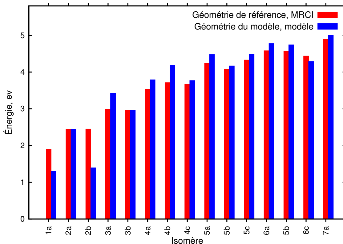
FIGURE A.4 – Comparaison des énergies de détachement de l'hydroxyde pour l'agrégat gelé entre calcul de référence MRCI et calcul avec le modèle classique décrivant \text{OH}^- en interaction avec un agrégat d'eau.
