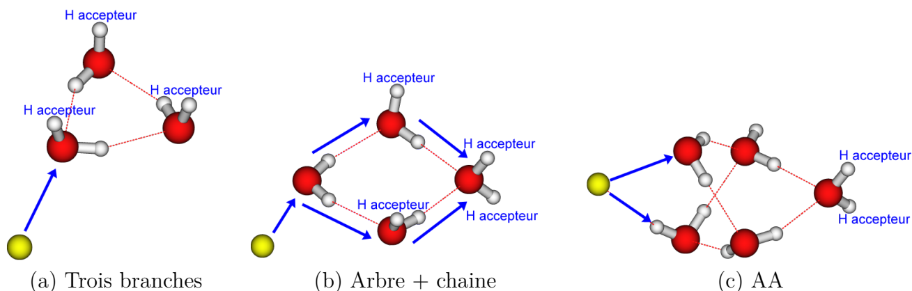
FIGURE 2.9 – Schéma présentant les trois grand motifs observé pour les agrégats \text{X}(\text{H}_2\text{O})_{n=1-7} ( \text{X}=\text{F} , \text{I} et \text{OH} ) pour les géométries minimisant l'énergie dans l'état triplet.
