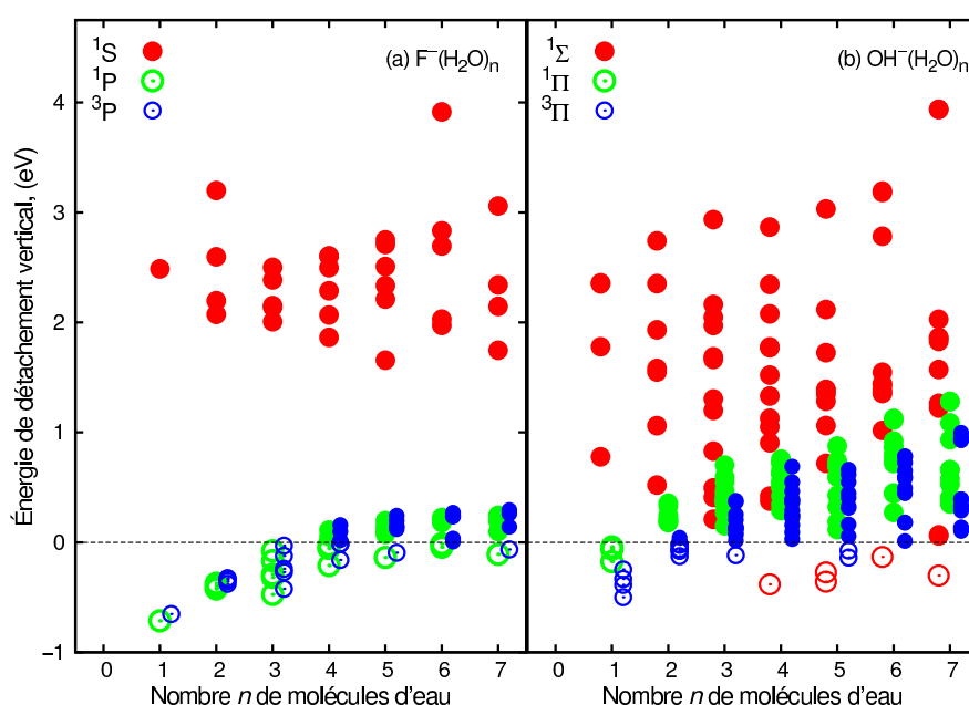
FIGURE 2.10 – EDV pour les états ^1S/^1\Sigma , ^1P/^1\Pi et ^3P/^3\Pi . Les symboles pleins correspondent aux isomères liés pour un état donné. Concernant le fluorure, les autres états P issues de la levée de dégénérescence par l’eau ne sont pas indiqués sur la figure par souci de clarté. Calcul effectué au niveau RASPT2, avec une base aug-cc-pVTZ.
