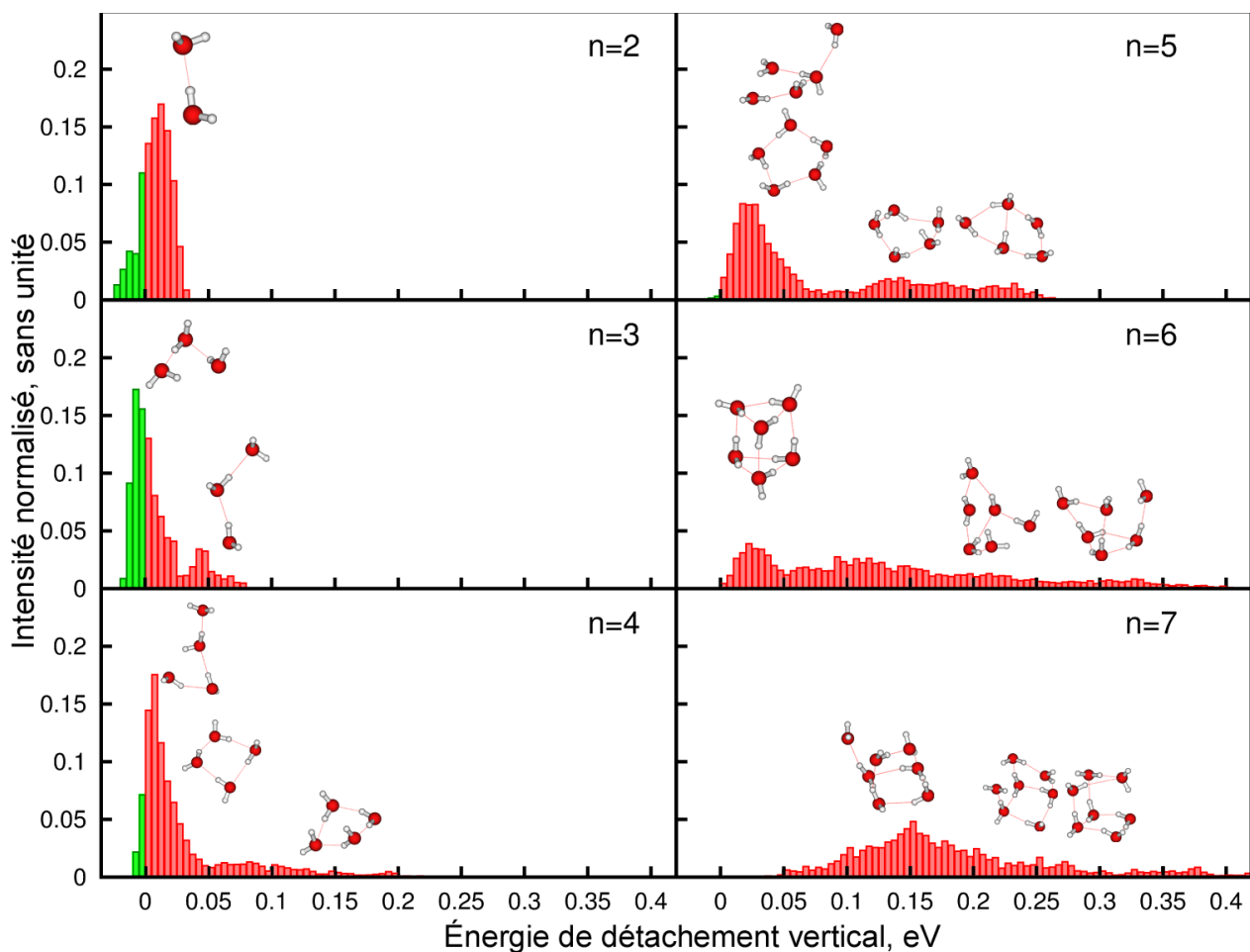
FIGURE 5.13 – Spectre en EDV de l'électron excédentaire pour (\text{H}_2\text{O})_{n=2-7}^- . Les barres en vert correspondent aux énergies pour lesquelles le système est censé s'ioniser spontanément de façon adiabatique. Pour les pics observés, des structures géométriques sont associées.
