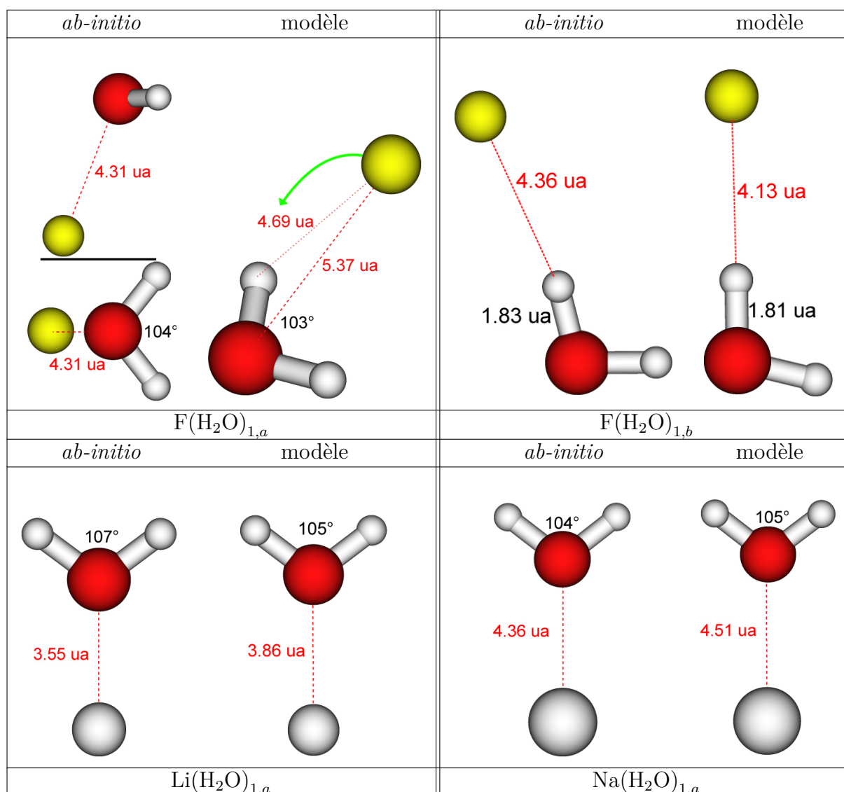
FIGURE 4.8 – Comparaison entre structures ab-initio et structures du modèle avec un soluté neutre à couche ouverte.
