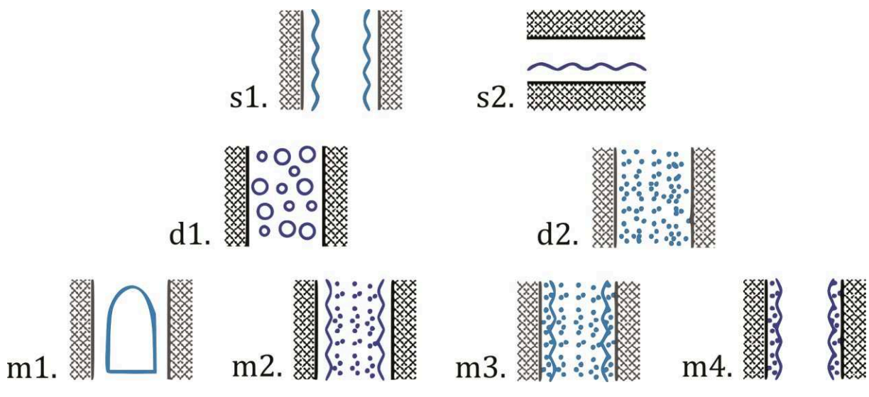
FIGURE 1.4 : Illustration des géométries d'écoulements diphasiques internes selon la classification de Ishii [23]. Ecoulements séparés : s1 . annulaire et s2 . film. Ecoulements dispersés : d1 . à bulles et d2 . à gouttes. Ecoulements mixtes : m1 . en bouchons, m2 . annulaire à gouttes, m3 . annulaire à gouttes et bulles et m4 . annulaire à bulles.
