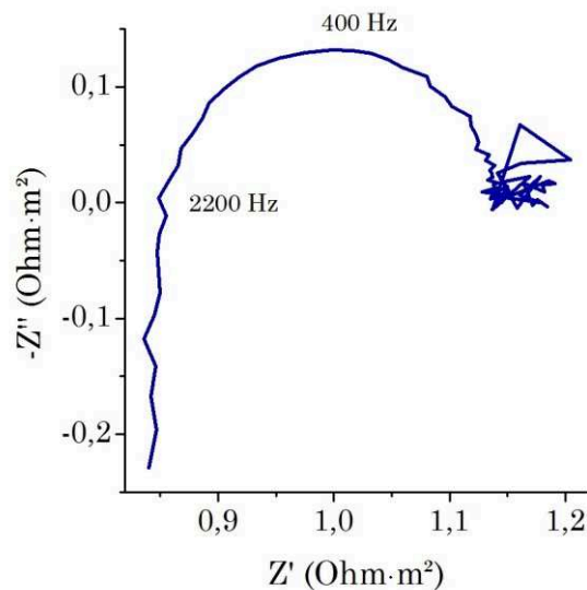
FIGURE 4.9 : Spectre d'impédance expérimental obtenu à j_{moy} = 690 A/m^2 et Re_{D_h} = 333 .
