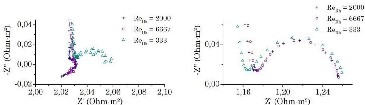
FIGURE 4.12 : Influence du débit d'électrolyte sur les impédances de bulles à j_{\text{moy}} = 173 \text{ A/m}^2 , (a) à gauche : valeurs mesurées et (b) à droite : valeurs simulées. Les courbes ont été déplacées sur l'axe des réels pour faciliter la comparaison.
