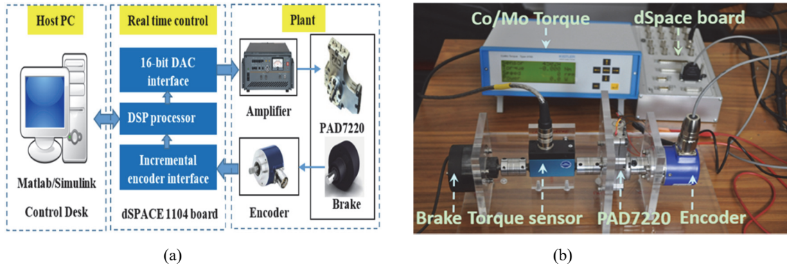
Fig.13. (a) Synoptique de système de positionnement de pad7220, (b) Plateforme expérimentale
