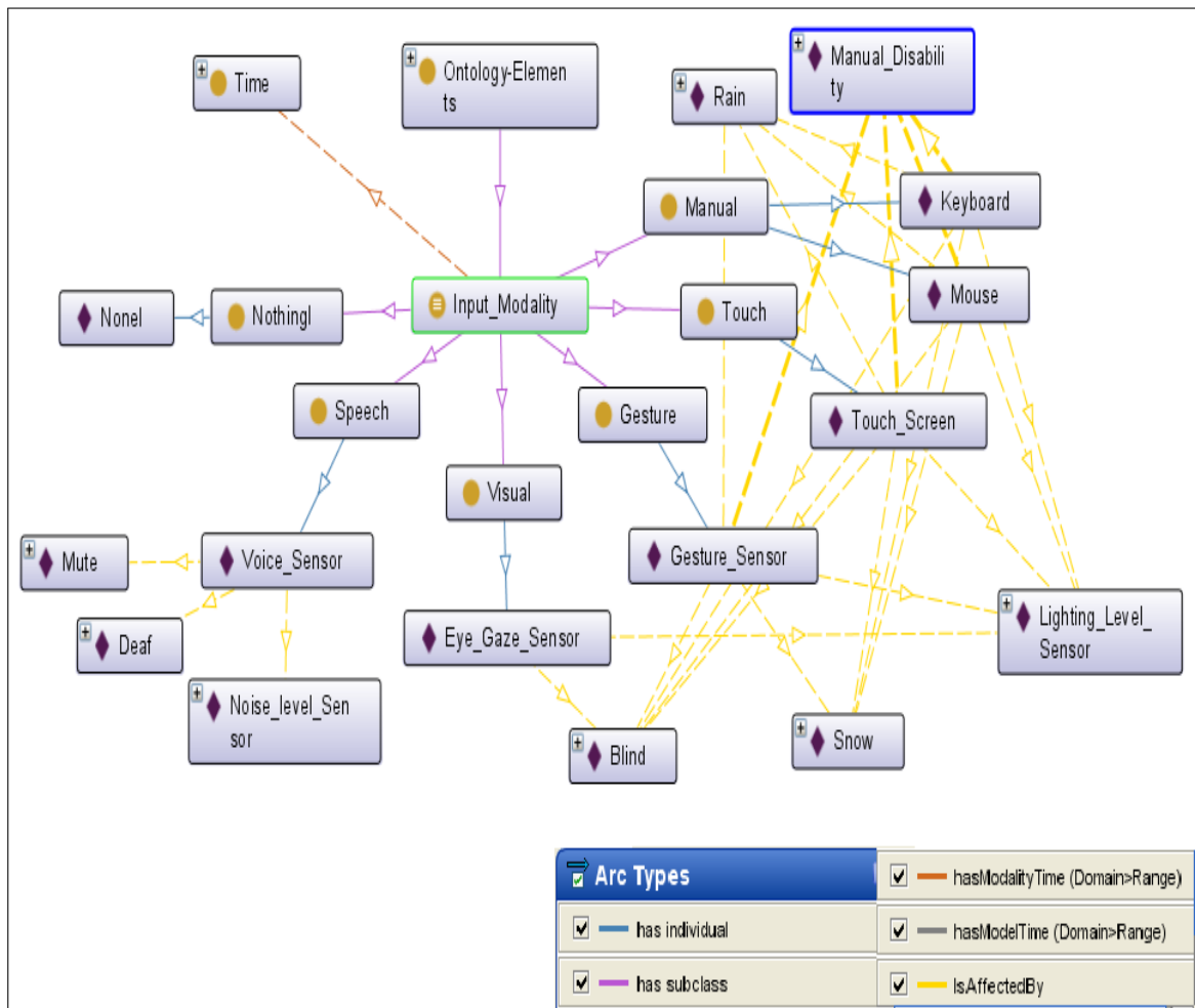
FIGURE 3.22: La classe “Input Modality”, ses sous classes et leurs individus
