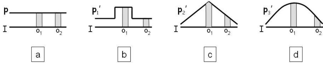
FIG. 5.6 – Distributions de probabilités (2D) : (a) uniforme, (b) par paliers, (c) linéaire, (d) non linéaire.
