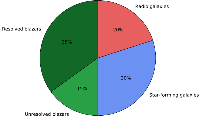
FIGURE 6.2 – À gauche : Répartition approximative de la contribution des différentes sources au fond gamma extragalactique entre 100 MeV et 820 GeV. À droite : Spectre de l'émission intégrée des blazars comparé au spectre du fond gamma extragalactique mesuré par Fermi /LAT (figure 3b, Ajello et al. 2015).
