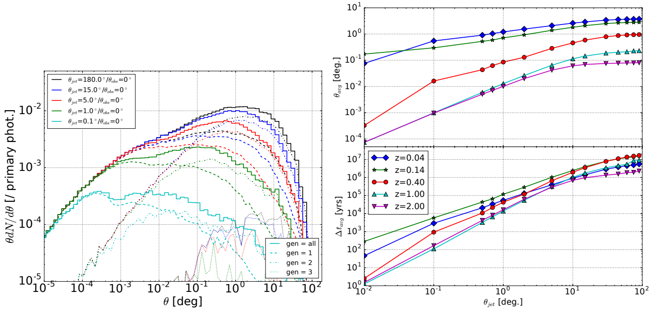
FIGURE 5.6 – À gauche : Distribution angulaire des photons (intégré en énergie et en temps) engendrée par la source standard décrite en préambule avec différents angles d’ouverture du jet \theta_{jet} ( 180^\circ étant une source isotrope). Les spectres sont normalisés à 1 photon émis. À droite : Angle moyen d’arrivée (haut) et temps moyen d’arrivée (bas) des photons avec une énergie supérieure à 1 GeV en fonction de l’angle d’ouverture du jet \theta_{jet} et pour différents redshifts z .
