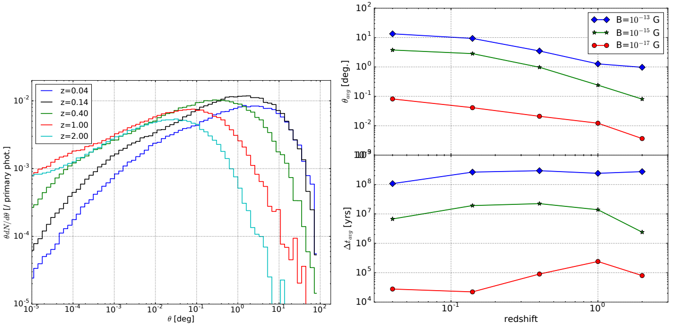
FIGURE 5.2 – À gauche : Distribution angulaire des photons (photons d'énergie supérieure à 1 GeV) engendrée par la source standard décrite en préambule et placée à différents redshifts z . Les distributions sont normalisées à 1 photon émis. À droite : Angle moyen d'arrivée (haut) et temps moyen d'arrivée (bas) des photons avec une énergie supérieure à 1 GeV en fonction du redshift z de la source et pour différentes amplitudes du champ magnétique extragalactique.
