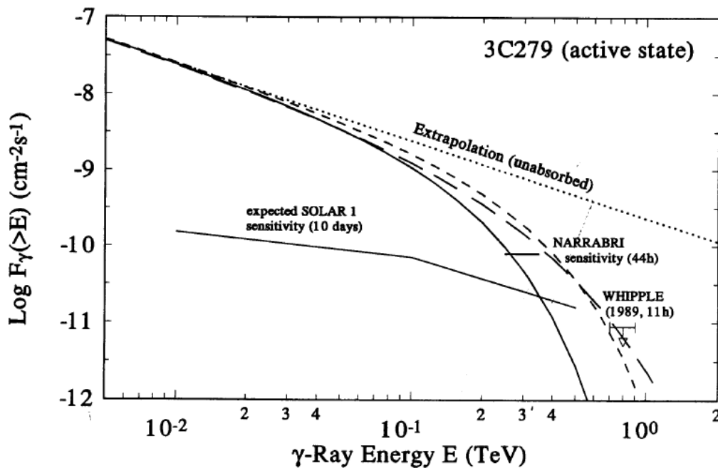
FIGURE 1.5 – Spectre supposé d'une source (pointillés) et spectres observés suite à la coupure due à l'absorption (Stecker et al. 1992).
