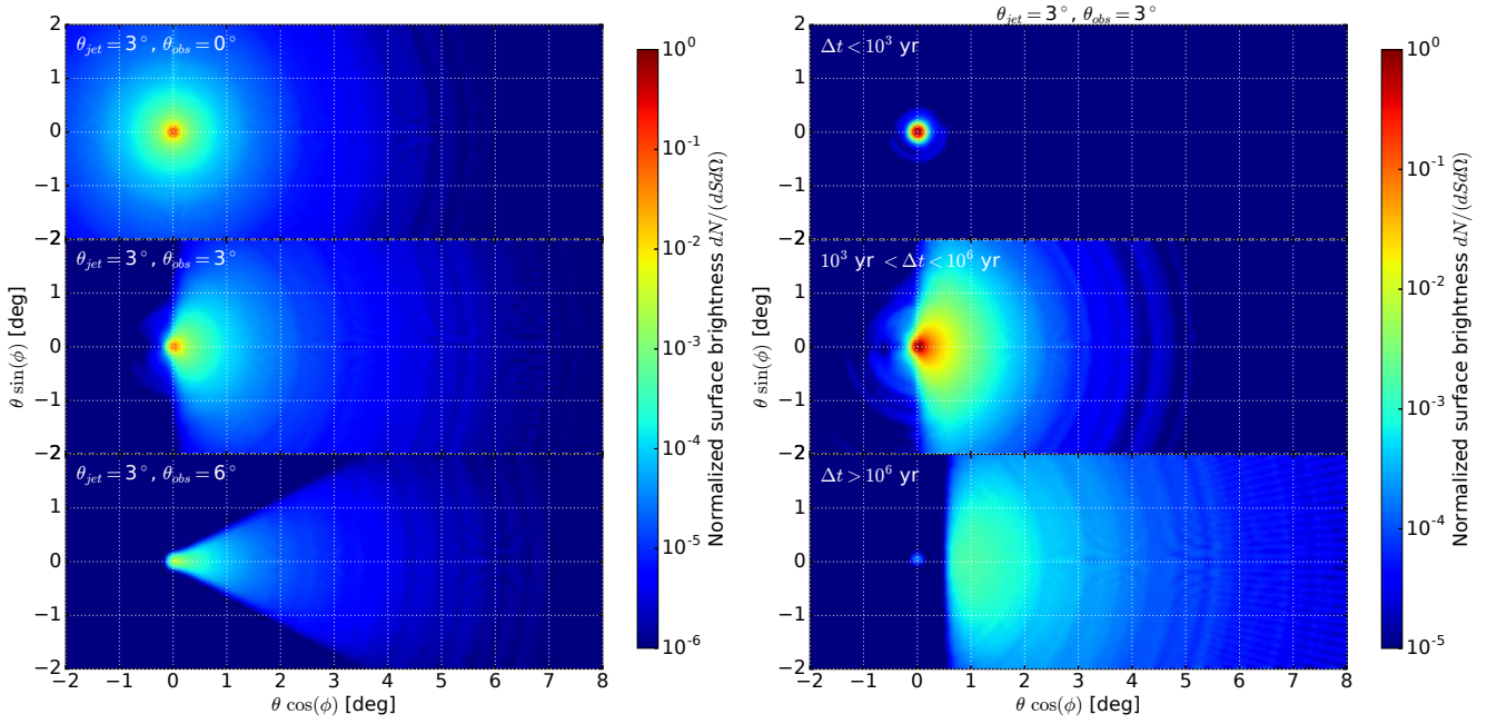
FIGURE 5.7 – Images de la source et de sa cascade pour une émission dans un jet d’ouverture \theta_{jet} = 3^\circ et différents désalignements du jet (à gauche) et pour une émission dans un jet d’ouverture \theta_{jet} = 3^\circ et un désalignement \theta_{jet} = 3^\circ observée dans une période de temps donnée après un burst par exemple (à droite, voir discussion section 4.2.3). L’échelle de couleurs a été normalisé sur l’émission maximale d’une source émettant dans la direction de l’observateur ( \theta_{obs} = 0^\circ ). Les photons sont sélectionnés avec une énergie supérieure à 1 GeV.
