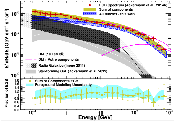
FIGURE 6.2 – À gauche : Répartition approximative de la contribution des différentes sources au fond gamma extragalactique entre 100 MeV et 820 GeV. À droite : Spectre de l'émission intégrée des blazars comparé au spectre du fond gamma extragalactique mesuré par Fermi /LAT (figure 3b, Ajello et al. 2015).
