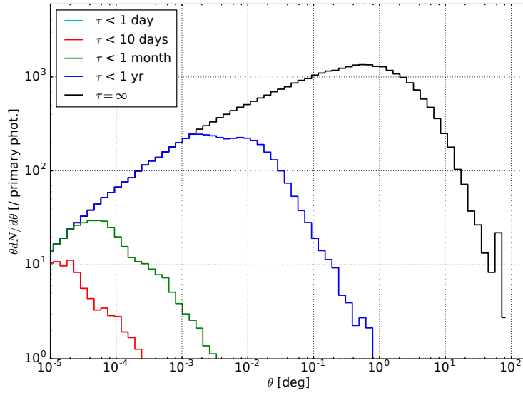
FIGURE 4.11 – Évolution temporelle de l'extension du halo d'une source mono-énergétique (100 TeV) située à 557 Mpc ( z = 0.13 ) ( B = 3 \times 10^{-16} G et E > 1 GeV). Composante du halo reçue après un certain temps \tau . \tau = 0 correspond à un photon source arrivé directement sans interaction.
