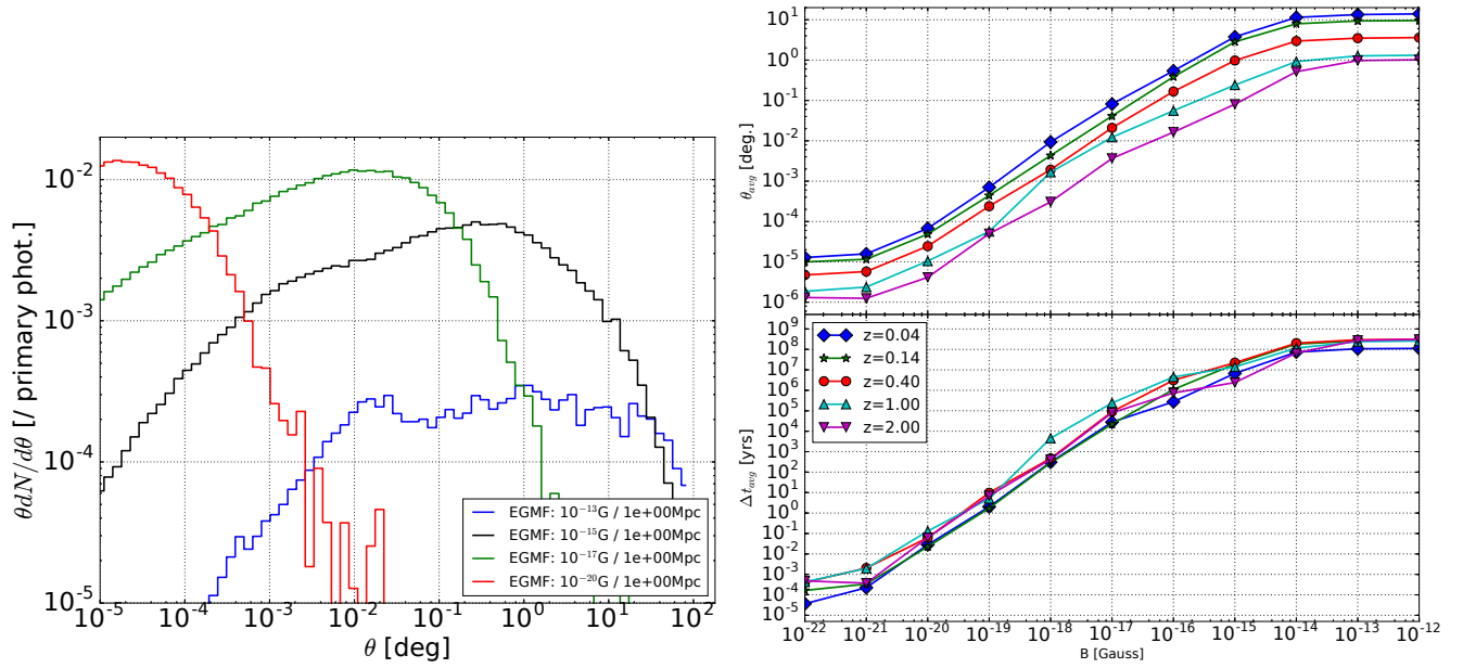
FIGURE 5.11 – À gauche : Distribution angulaire des photons (intégré en énergie et en temps) engendrée par la source standard décrite en préambule pour différentes amplitudes du champ magnétique extragalactique. Les spectres sont normalisés à 1 photon émis. À droite : Angle moyen d'arrivée (haut) et temps moyen d'arrivée (bas) des photons avec une énergie supérieure à 1 GeV en fonction de l'amplitude du champ magnétique extragalactique et pour différents redshifts z .
