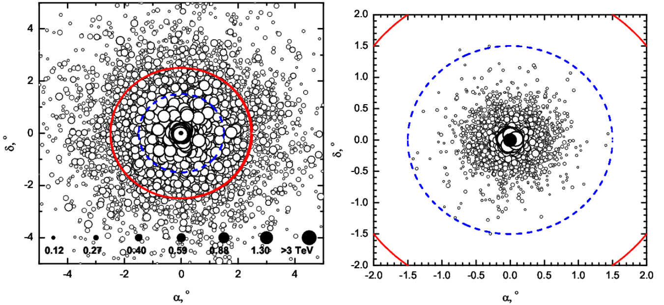
FIGURE 1.11 – Deux images du halo de paires pour un champ magnétique extragalactique de respectivement 10^{-14}\text{G} et 10^{-15}\text{G} . En tiret bleu est le champ de vue de MAGIC ( 1.5^\circ ) et en rouge le champ de vue de H.E.S.S. ( 2.5^\circ ) (Elyiv et al. 2009).
