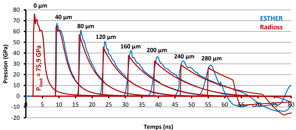
Figure 61 - Propagation et amortissement hydrodynamique d'une impulsion de pression dans une cible de Cuivre ( 2,920 \text{ TW/cm}^2 , soit P_{load} = 75,9 \text{ GPa} ), simulée sous ESTHER (en bleu) et sous Radioss (en rouge). Les profils de pression sont extraits tous les 40 \mu\text{m}
