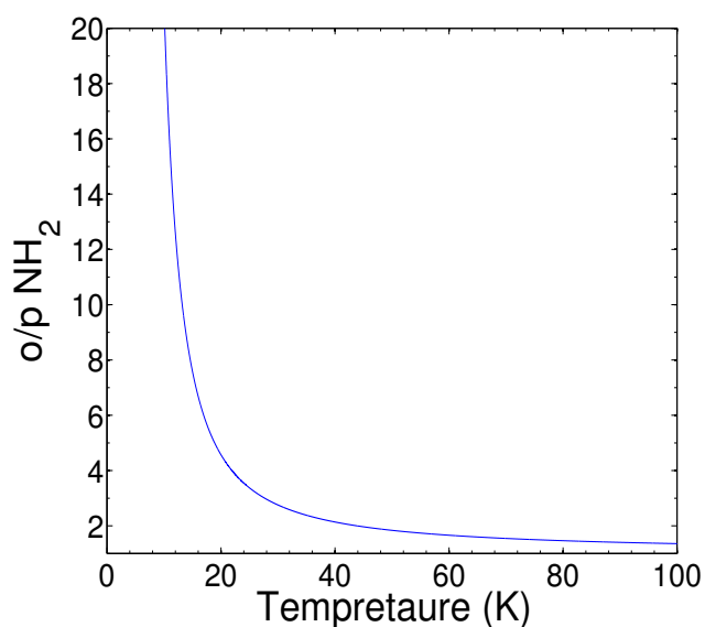
FIGURE VI.11: Évolution du \text{ROP}(\text{NH}_2) à l'équilibre thermodynamique en fonction de la température.
