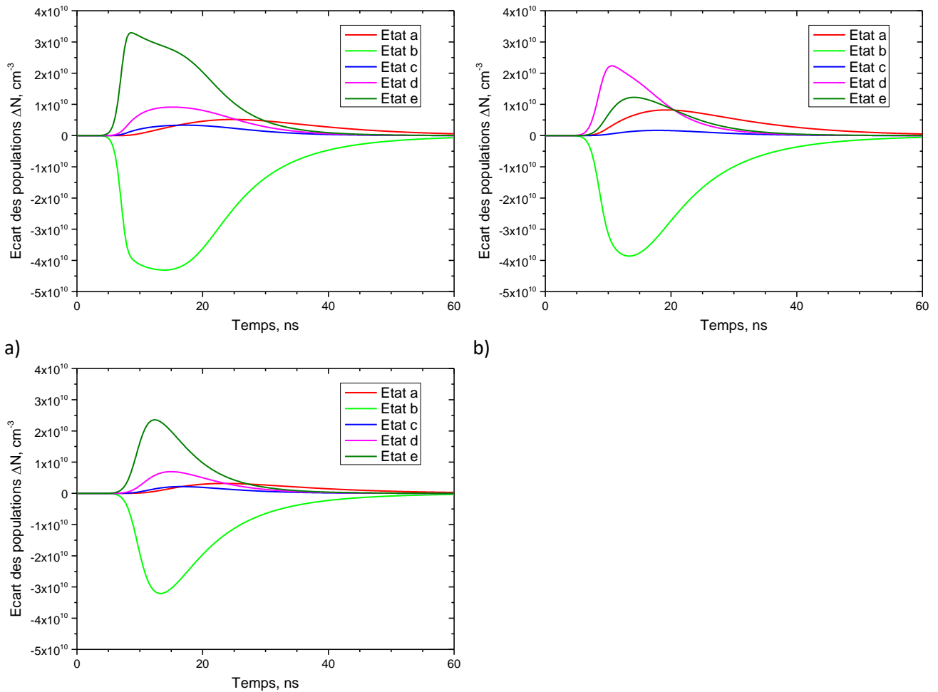
Figure 3.45 Variation de la densité de population des états en fonction du temps ; I_{\text{theo}} = 15 \text{ kW.cm}^{-2} , P = 53 \text{ mbar} ( \text{N}_2 ), T=1200 \text{ K} . Le laser est centré sur a) 309,3606 nm, b) 309,3737 nm, c) 309,3636 nm
