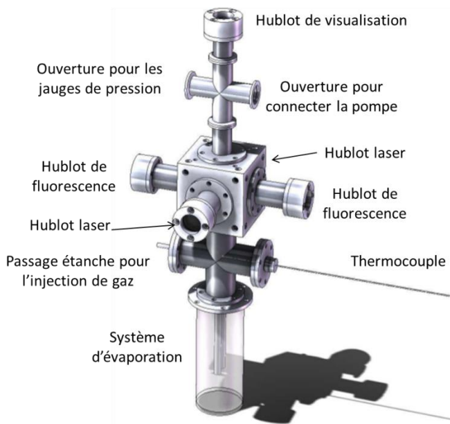
Figure 2.5 a) Dessin CAO de l'enceinte; b) Photo de l'enceinte
