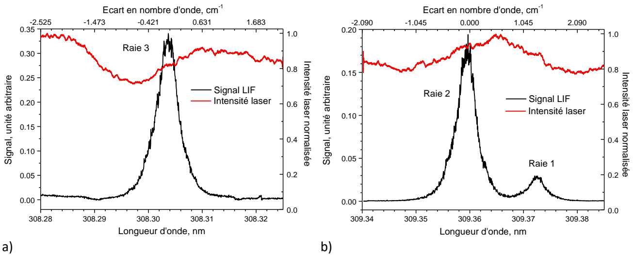
Figure 3.19 Exemple de profils spectraux enregistrés dans N_2 à 53 mbar et T=1200 K avec une intensité laser de 70-100 \text{ W.cm}^{-2} : a) Raie 3 ; b) Raies 1 et 2. La fluorescence est détectée à résonance. L'intensité laser (en rouge) est également enregistrée
