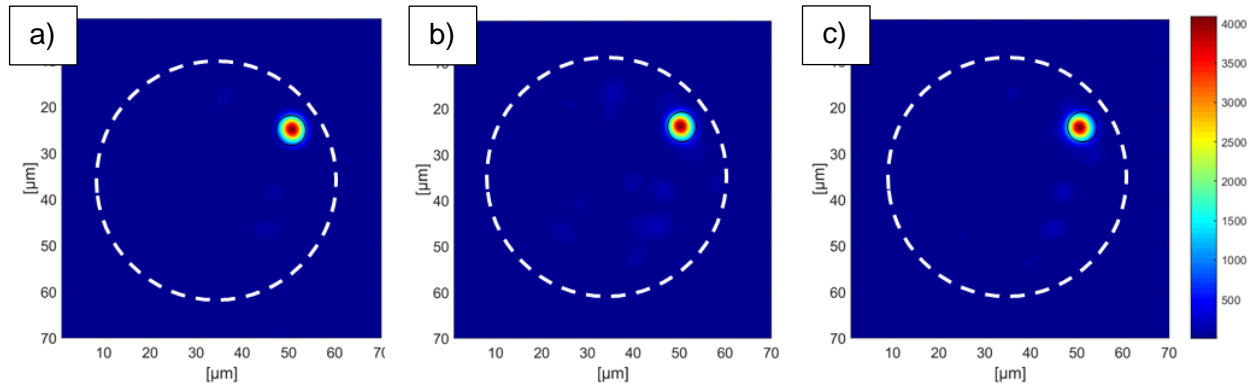
Figure III-24 : Résultats expérimentaux de la focalisation excentrée à travers la fibre multimodale amplificatrice pompée avec une puissance de 40 W : éclairage en extrémité de fibre a) après optimisation en régime de gain petit signal (24,5 dB), b) lorsque l'optimisation est effectuée en régime petit signal et l'enregistrement pris après augmentation de la puissance signal jusqu'au régime de saturation de gain (10,3 dB), c) après optimisation en régime de saturation de gain (10,3 dB)
