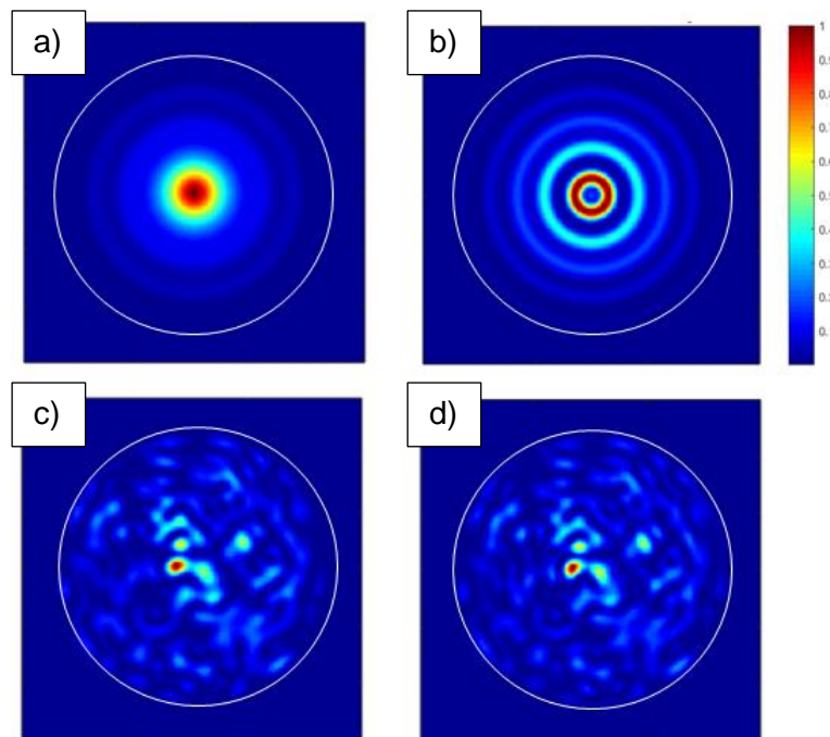
Figure III-22 : Eclaircements en extrémité de FMM obtenus numériquement, a) avec un front d'onde excitateur plan et en régime d'amplification petit signal b) avec un front d'onde excitateur plan et en régime de saturation de gain. c) avec un front d'onde excitateur structuré aléatoirement et en régime d'amplification petit signal d) avec un front d'onde excitateur structuré aléatoirement et en régime de saturation de gain
