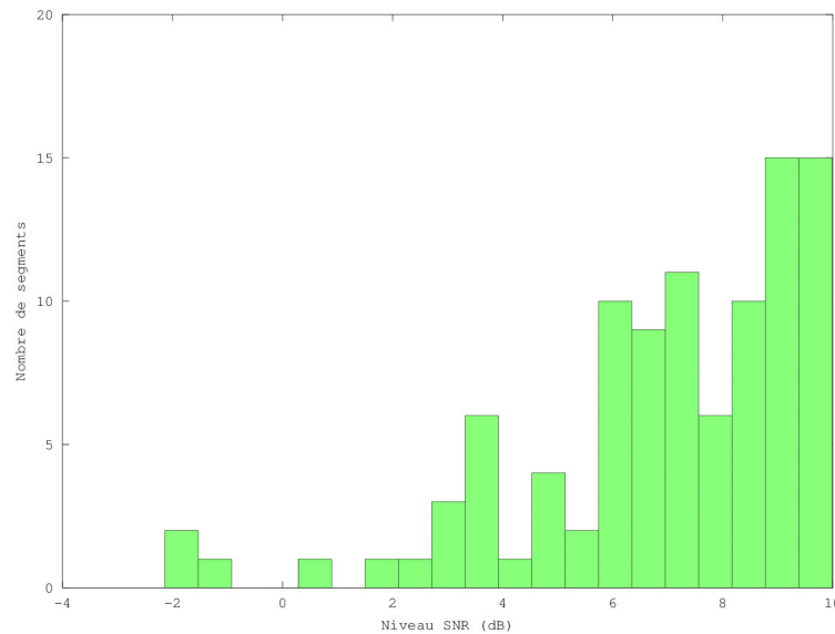
FIGURE 4.3 – Histogramme des niveaux de SNR des segments de l'ensemble I.
