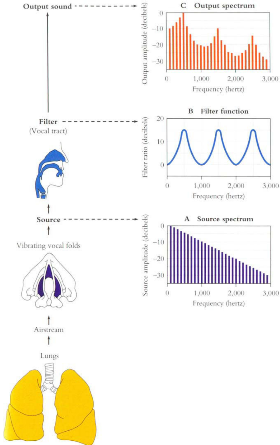
FIGURE 1.3 – Aperçu détaillé du modèle source-filtre (source : http://www.ling.upenn.edu/courses/Spring_2001/ling001/phonetics.html ).
