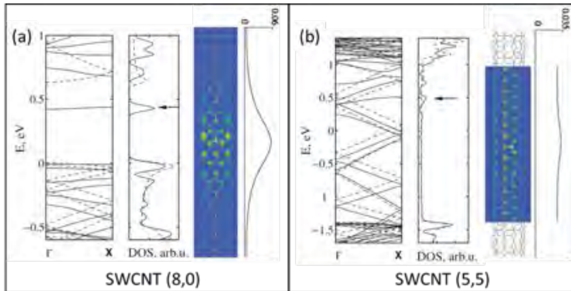
Figure 2.10 Structure de bandes, densité d'états électroniques et densité de spin d'un SWCNT (8,0) à gauche et d'un SWCNT (5,5) à droite. Les lignes solides correspondent au CNT dopé par de l'azote en configuration graphitique et les lignes en pointillés au CNT original. Les flèches indiquent l'état du dopant [Nevidomskyy et al., 2003].
