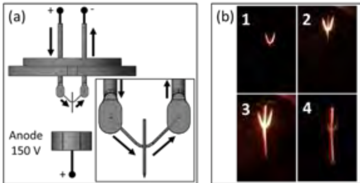
Figure 4.5(a) Configuration schématique du banc de flash. Les flèches indiquent le flux de courant dans la cathode pendant le flash. (b) Images extraites d'une vidéo de flash ( 120 \text{ fps} )
