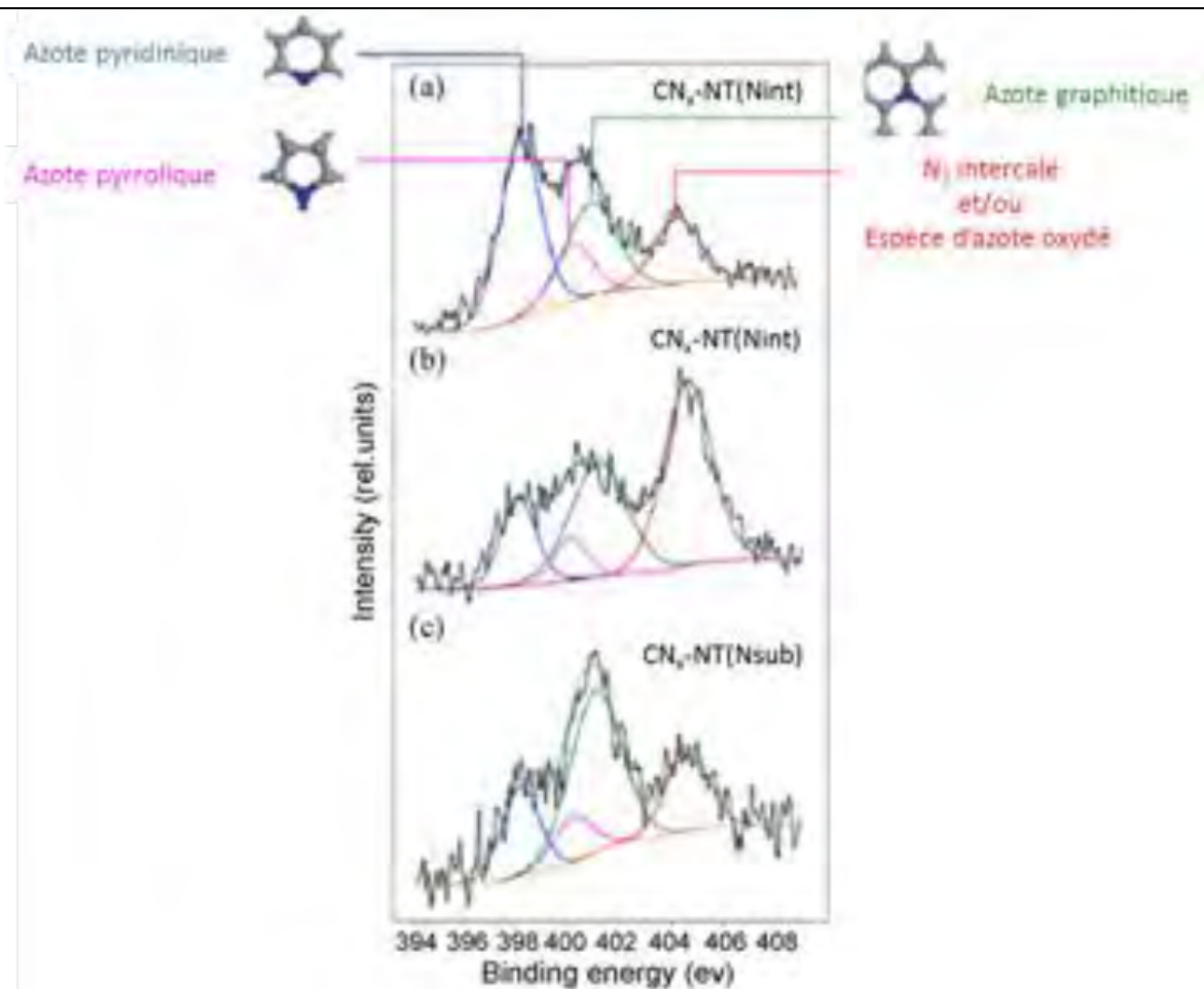
Figure 2.18 Spectres XPS d'échantillons synthésés à 650°C (a), 750°C (b) et 850°C (c) [Chizari et al., 2010].
