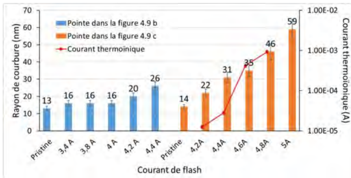
Figure 4.9 Variation du rayon de courbure de l'apex après différents traitements flash. La courbe rouge correspond au courant thermoionique détecté pendant le flash.
