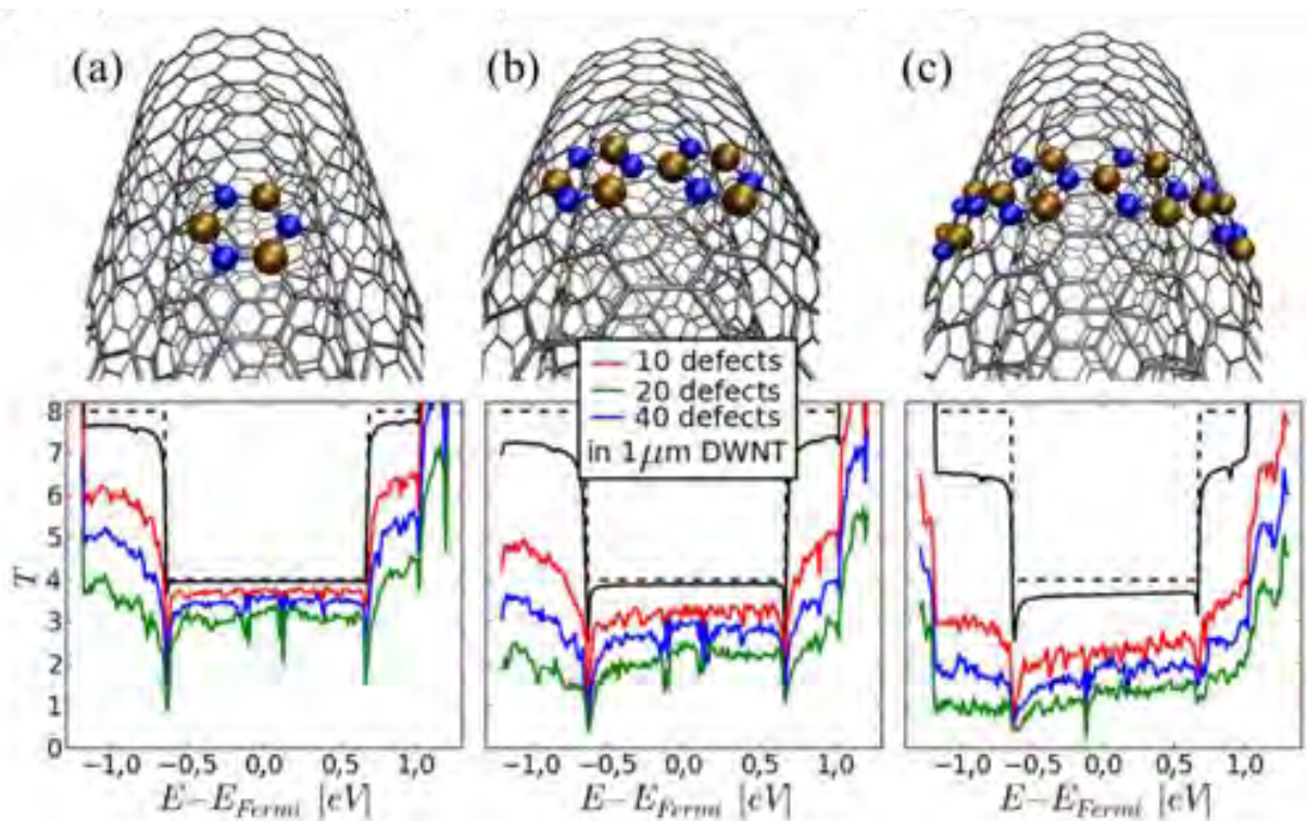
Figure A.1 Les figures du haut illustrent les différentes configurations de nano-domaines de BN incorporés dans le réseau hexagonal de la paroi extérieure d'un NT de carbone. Les figures du bas montrent les courbes de conductance quantiques en fonction du nombre de ces « défauts » qui sont distribués au hasard dans un DWNT de carbone de 1 \mu\text{m} de long suivant la nomenclature suivante : DWNT pur (ligne en pointillé noire), 1 défaut (ligne solide noire), 10 défauts (ligne solide rouge), 20 défauts (ligne solide verte) et 40 défauts (ligne solide bleue).
