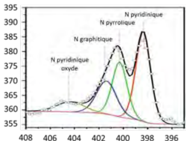
Figure 2.22 Spectre XPS des CN_x -NTs traités avec NH_3 à 800\text{ }^\circ C [Nagaiah et al., 2010].
