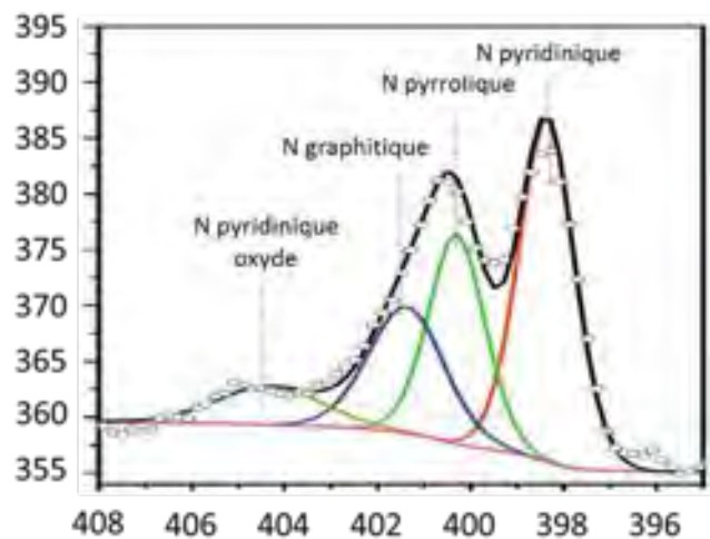
Figure 2.22 Spectre XPS des CN_x -NTs traités avec NH_3 à 800\text{ °C} [Nagaiah et al., 2010].
