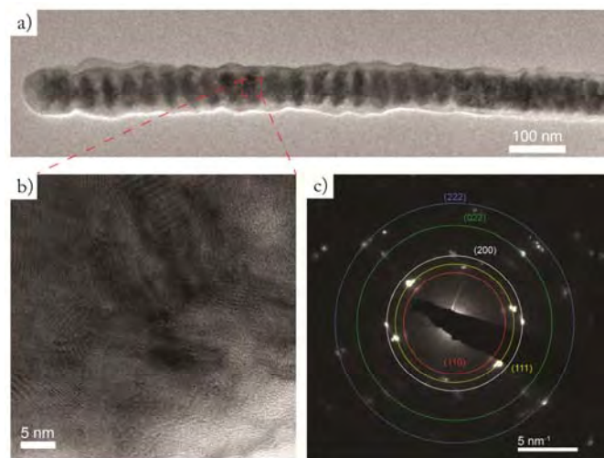
Figure 10 a) Image en champ clair d'un nanofile Co/ Cu (25nm/15nm), b) image MET haute résolution, c) cliché de diffraction d'une zone de cobalt
