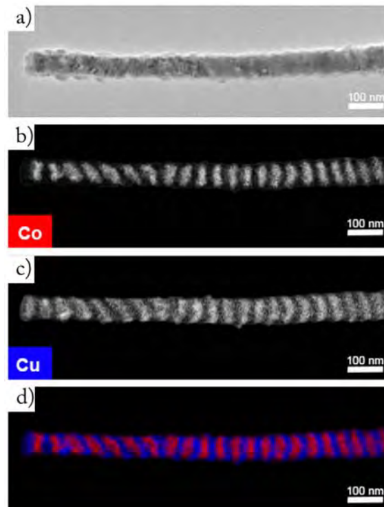
Figure 11 a) Image en champ clair d'un nanofil Co/Cu (25nm/15nm), b) cartographie du cobalt, c) cartographie du cuivre, d) superposition des deux cartographies
