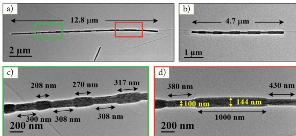
Figure 16. Images MET champ clair de deux fils FeCoCu à diamètre modulé de a) 13\ \mu\text{m} et b) de 4,7\ \mu\text{m} de longueur. Les diamètres des nanofils et les longueurs de segments sont mesurés à partir des images à fort grandissement en MET correspondant aux zones rectangulaires en a). c) et d) illustrent le changement progressif de la longueur des segments.
