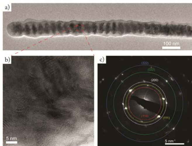
Figure 10 a) Image en champ clair d'un nanofil Co/Cu (25nm/15nm), b) image MET haute résolution, c) cliché de diffraction d'une zone de cobalt
