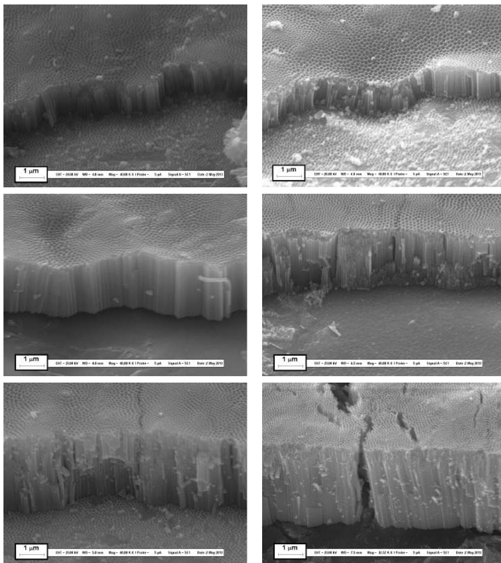
Figure 97 – Morphologie MEB d'électrodes de 3 \text{ cm}^2 (colonne de gauche) ou de 24 \text{ cm}^2 (colonne de droite) avec des charges d'anodisation de 2 \text{ C/cm}^2 (ligne du haut), 4 \text{ C/cm}^2 (ligne du milieu) et 6 \text{ C/cm}^2 (ligne du bas).
