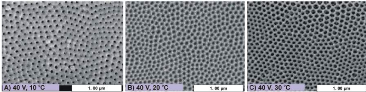
Figure 17 – Synthèse de nanotubes à différentes températures réalisée dans un électrolyte de 3ème génération comprenant de l'éthylène, du \text{NH}_4\text{F} (0,38 % en masse) et de l'eau (1,79 % en masse) [110].
