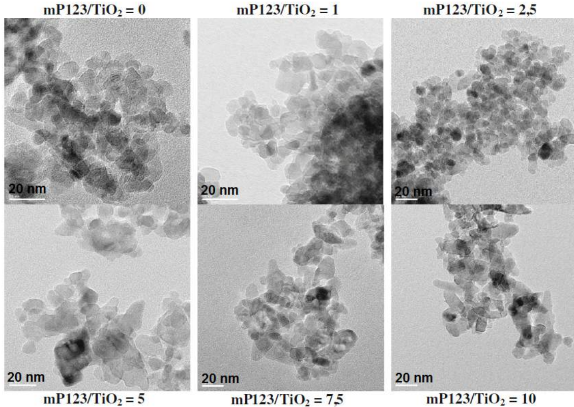
Figure 53 – Analyse TEM des nanoparticules de TiO 2 synthétisées en présence de P123.
