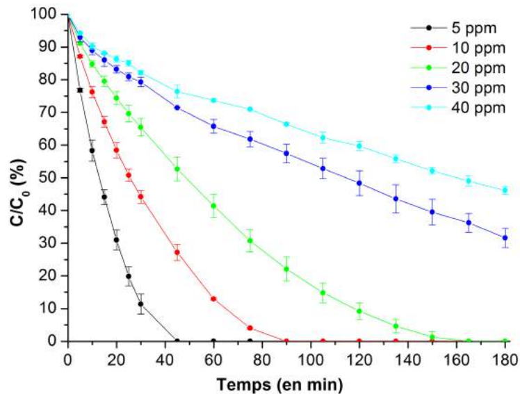
Figure 67 – Influence de la concentration initiale en paraquat sur la cinétique de dégradation avec 6 lampes UV-C et un volume à traiter de 1 litre.
