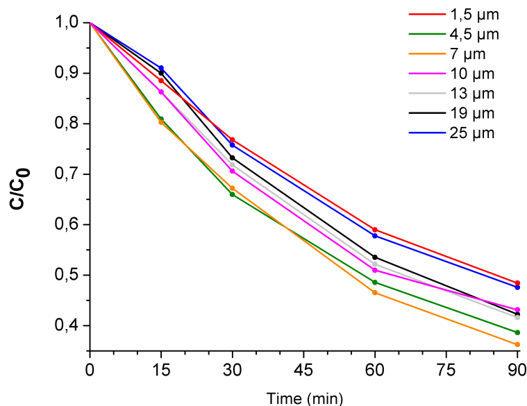
Figure 88 – Dégradation photocatalytique du paraquat dans la cellule en quartz avec les nanotubes de \text{TiO}_2 de différentes longueurs.
