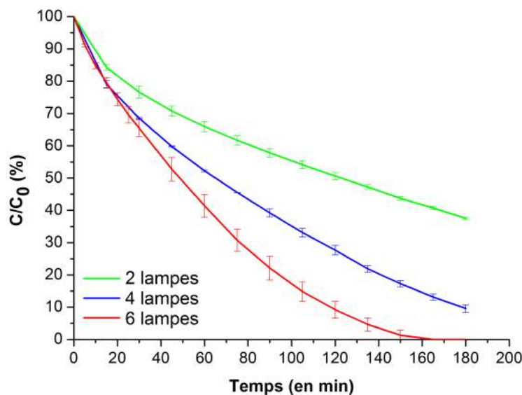
Figure 62 – Cinétique de dégradation photocatalytique du paraquat avec un nombre variable de lampes tubulaires UV-C 8W ( [\text{Paraquat}]_{t=0\text{min}} = 20 ppm, V = 1 l).
