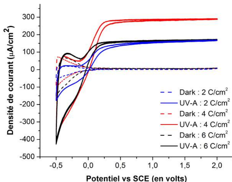
Figure 104 – Etude voltampérométrique d'électrodes en nanotubes de TiO 2 /Ti synthétisés avec une charge d'anodisation de 2 C/cm 2 (L = 1,6 µm), 4 C/cm 2 (L = 3,2 µm) ou 6 C/cm 2 (L = 5,6 µm) dans un électrolyte Na 2 SO 4 0,1 M.
