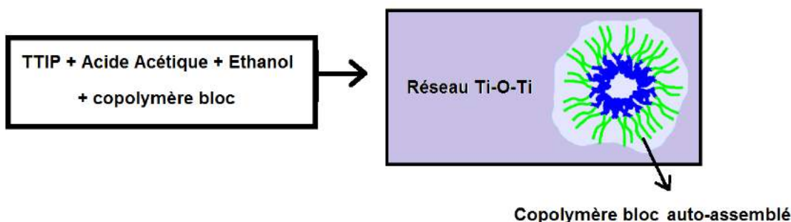
Figure 14 – Formation de mésopores par incorporation d'un copolymère bloc dans la synthèse sol-gel.
