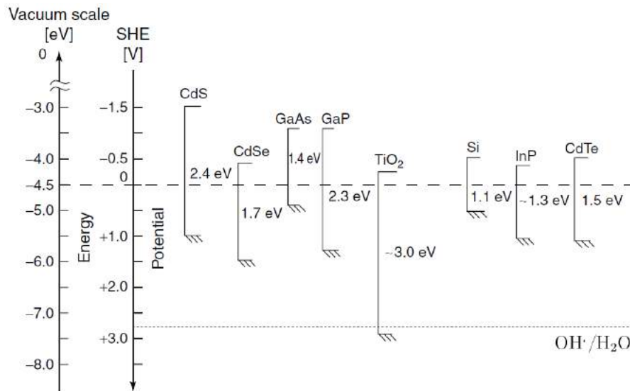
Figure 5 – Représentation de la position des bandes de différents semiconducteurs par rapport à l'échelle du vide [36].
