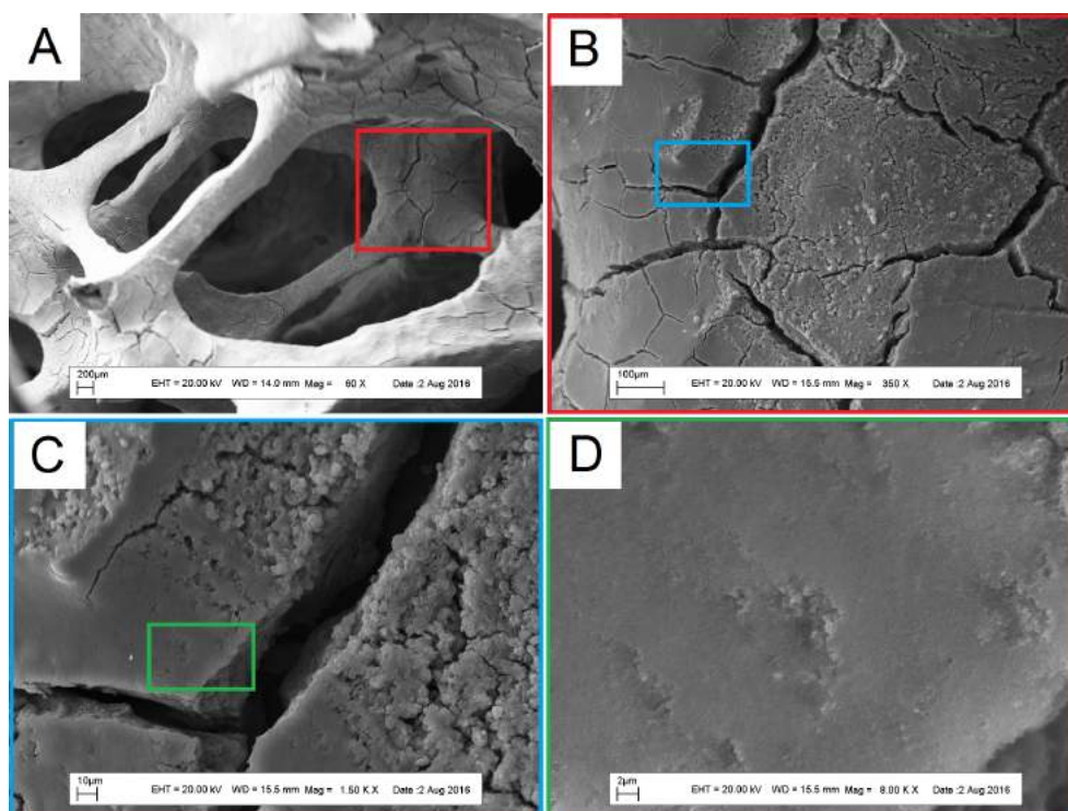
Figure 61 – Images MEB des mousses recouvertes de TiO 2 P25.
