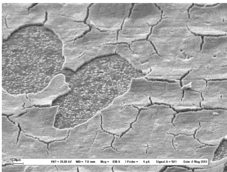
Figure 81 – Image MEB de nanotubes peu adhérents à la surface du titane.
