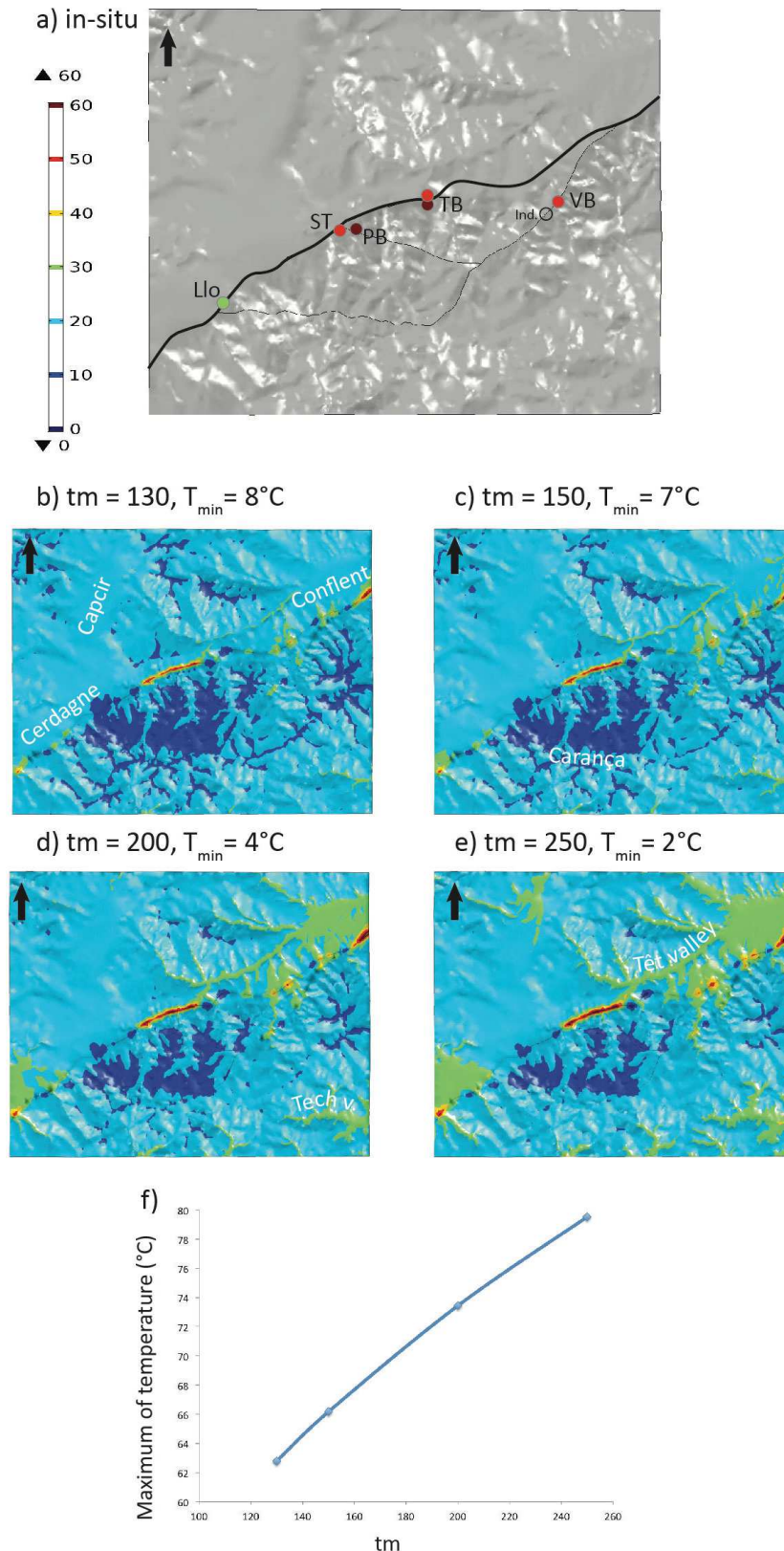
FIGURE 44: Etude paramétrique du coefficient tm ( k_f = 7.10^{-15} \text{ m}^2 , k_f = 10^{-16} \text{ m}^2 , T_{ext} = 20^\circ\text{C} ) (échelle des températures commune pour a-e). A) Distribution et températures des sources hydrothermales observées sur le terrain ( in-situ ) de la vallée de la Têt. B, C, D, E : la distributions des anomalies de températures, des sources hydrothermales et les températures d'infiltration des fluides sur les reliefs ( T_{min} ) pour différentes valeurs de tm . F) Températures maximales des sources hydrothermales en fonction de tm .
