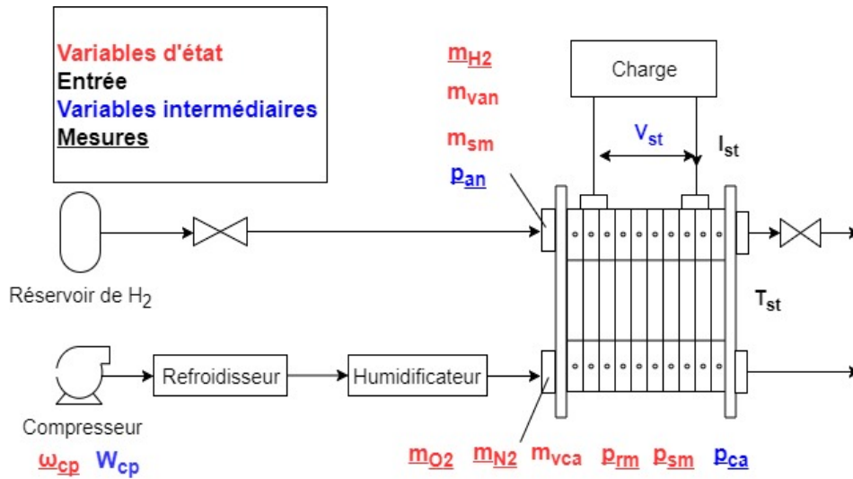
FIGURE 4.3 – Modèle d'une pile à combustible
