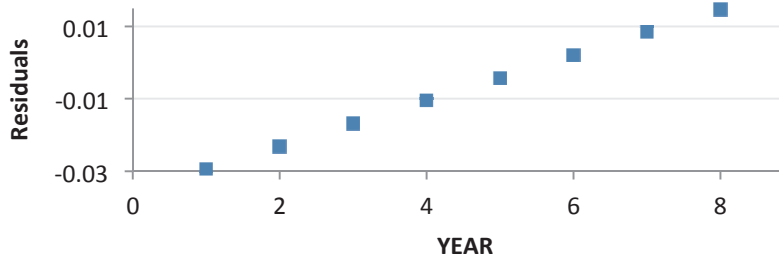
Weibull regression parameters
