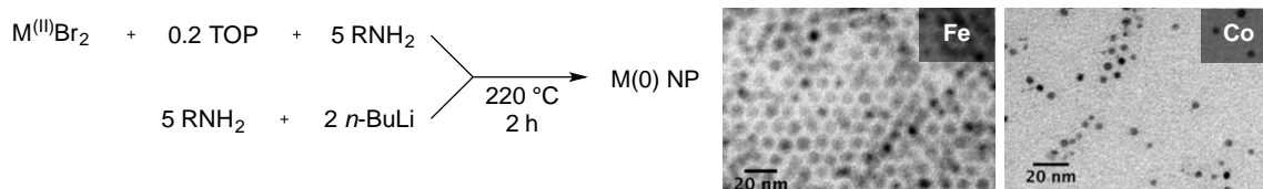
Figure R-11. Méthode « deux pot »: NPs Fe ( D = 6,8 \pm 0,8 nm) et Co ( D = 4,5 \pm 0,6 nm) dérivées de MBr_2 pré-mélangées avec 5 équiv. oléylamine, ajoutée à un mélange de 2 équiv. n -butyllithium avec 5 équiv. oléylamine supplémentaires, chauffée à 220 °C pendant 2 h.
