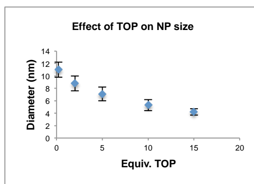
Figure R-3. Formation de NPs Ni de la décomposition du nickel(II) dioleamide en NPs Ni(0) dans le toluène avec des quantités variables de TOP.
