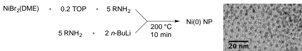
Figure R-6. \text{NiBr}_2(\text{DME}) pré-mélangé avec 5 équiv. oléylamine et 0,2 équiv. TOP, ajouté au mélange de 2 équiv. N-butyllithium avec 5 équiv. oléylamine de plus, chauffée à 200 \text{ }^\circ\text{C} pendant 10 min. ( D = 3,0 \pm 0,6 nm).
