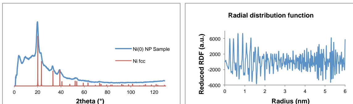
Figure R-5. Gauche: Diffractogramme WAXS de NPs Ni(0) montrés dans Figure R-4. Droite: Fonction de répartition radiale (RDF) des particules, révélant la taille des zones cristallines.
